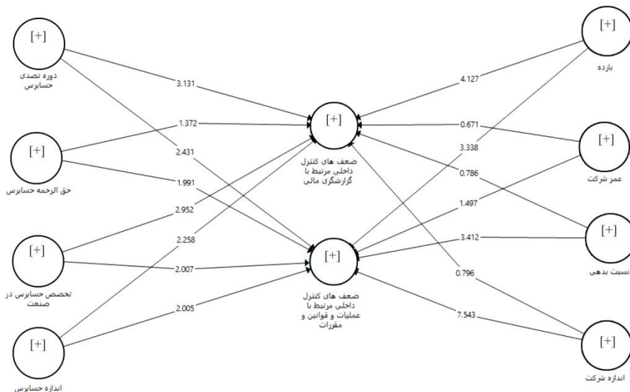
شکل ۱. مقادیر آماره t برای مدل مربوط به مسیر متغیرهای مستقل به متغیرهای واسطه‌ای
