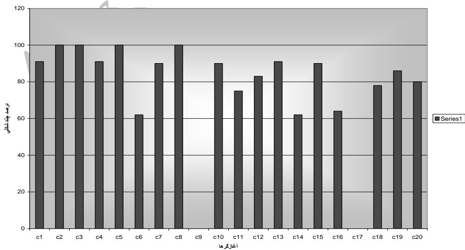
شکل ۲- نمودار درصد چند شکلی برای آغازگرها
