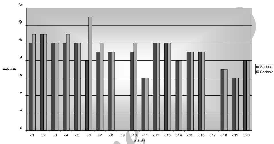
شکل ۱- نمودار مربوط به تعداد باندهای تکثیر شده و باندهای چندشکل بزاء هر آغازگر
