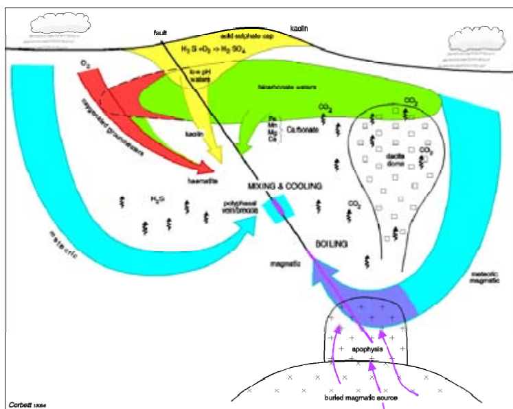
شکل ۱۳. سیالات هیدروترمالی منشأ گرفته از توده نفوذی و تزریق پی در پی آن در گسل‌های منطقه و اختلاط با آبهای جوی و تهنشینی شدن ماده معدنی [۴۲].
