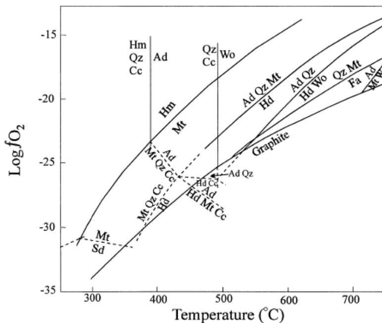
شکل ۳. نمودار در \log fO_2 در فشار ۵۰۰ بار و X_{CO_2}=0.1 برای سیستم Ca-Fe-Si-C-O-H (Einaudi, 1982) Ad=andradite, Cc=calcite, Fa=fayalite, Hd=hedenbergite, Hm=hematite, Mt=magnetite, Qz=quartz, Sd=siderite and Wo=wollastonite.
