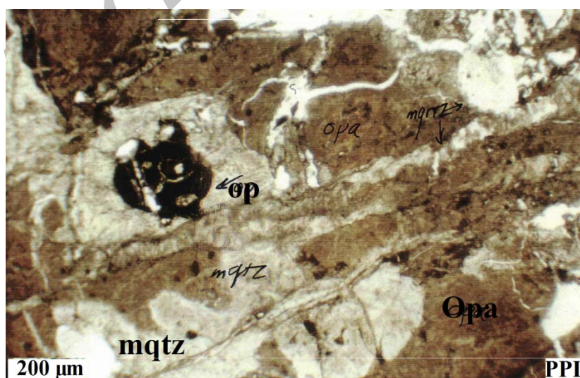
شکل ۷. تصویر میکروسکوپی یک نمونه لیستونیت سیلیسی برداشته شده از مجاورت رگه سینابر، حاوی کانیهای کلسدونی (کوارتز میکروکریستالین: mqtz)، اوپال (opa) و اوپاک (op). کانی اوپاک در این نمونه سینابر است.
