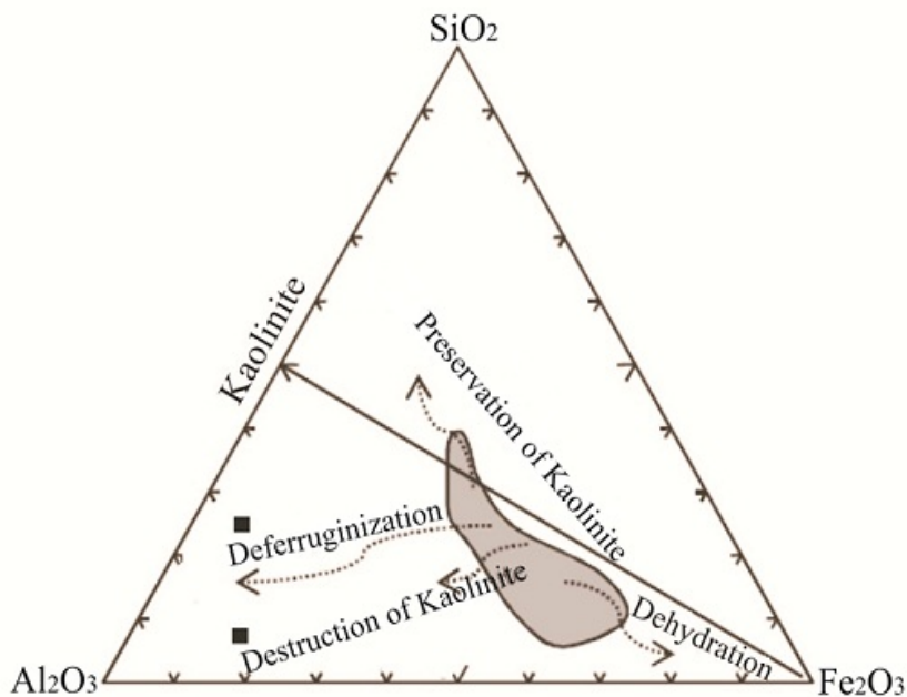
شکل ۱۰. نمودار مسیر زمین‌شیمیایی برگرفته از [۳۸] نشان‌دهنده روندهای مختلف فرآیندهای بوکسیتی‌زایی است. در این جا مسیر سایه‌زده شده بیانگر داده‌های منطقه آهن‌دار می‌باشد [۳۹]. نمونه‌های بوکسیتی منطقه تحت تأثیر تخریب کائولینیت و آهن‌زدایی قرار گرفته‌اند.
