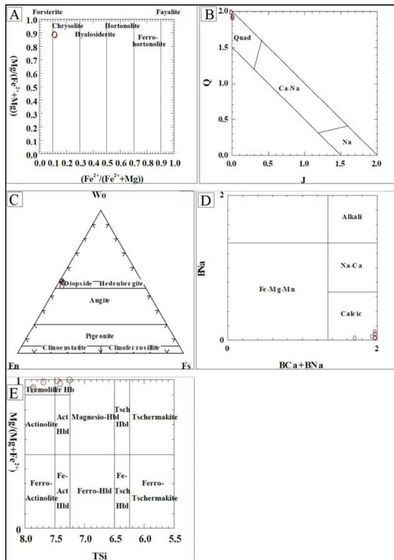
شکل ۶. A: نمودارهای ترکیب شیمیایی کانیهای الیوین، B و C: کلینوپیکروکسن، D و E: آمفیبول موجود در رلیت‌های افیولیت ناین (نمودارها برگرفته از (Deer et al., 1992)).
