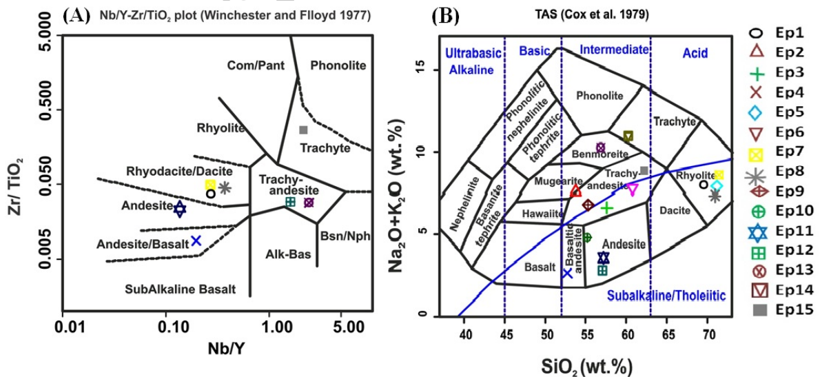
شکل ۱۴. رده‌بندی سنگهای منطقه اسفوردی با استفاده از A: نمودار وینچستر و فلوید، B: نمودار (TAS) (Winchester and Floyd, 1977)؛ B: نمودار (TAS) (Cox et al., 1979)
