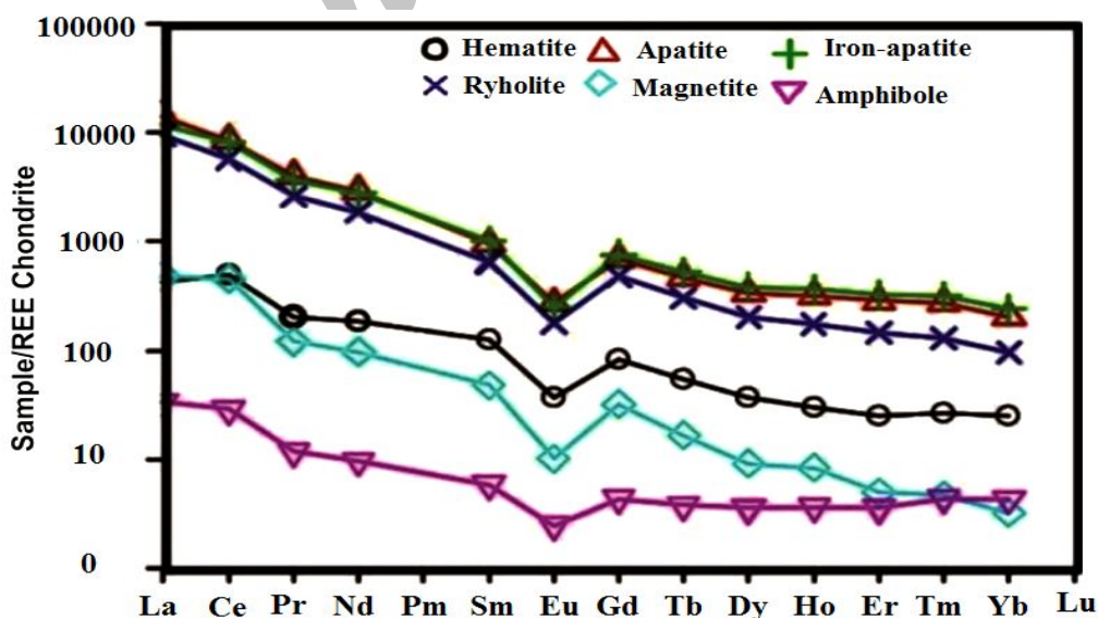
شکل ۱۶. الگوی به‌هم‌نگار شده توزیع عناصر نادر خاکی در انواع کانسنگ و سنگهای درون‌گیر در کانسار اسفوردی (داده‌های کندریت از (Boynton, 1985)).
