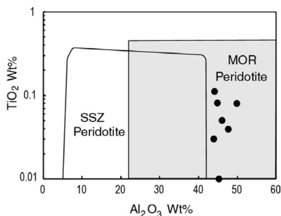
شکل ۱۴. نمودار TiO 2 (درصد وزنی) در مقابل Al 2 O 3 (درصد وزنی) در اسپینل‌ها برای شناسایی محیط زمین‌ساختی هارزبورگیت‌های کمپلکس دگرگونی شرقی خوی. محدوده‌های زون بالای فروانش و پشته میان اقیانوسی از کامنتسکی و همکاران (Kamenetsky et al., 2001)
