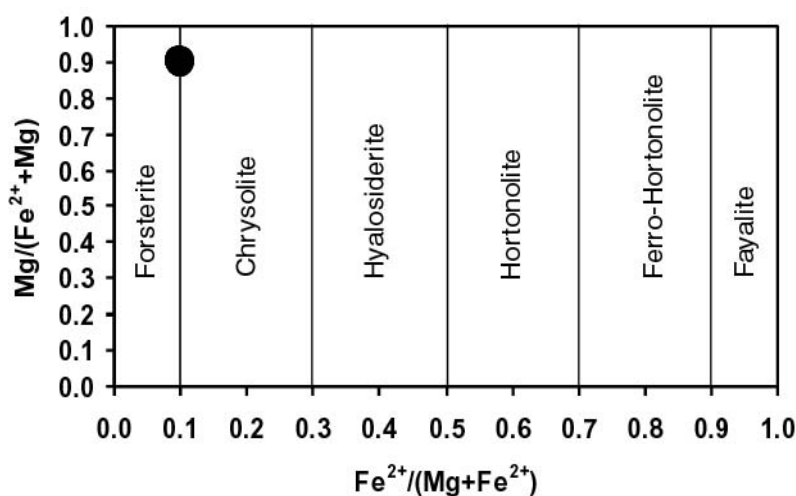
شکل ۳. ترکیب اولیوین‌ها در هارزبورگیت کمپلکس دگرگونی شرقی خوی در نمودار Fo-Fa از ریچارد (Richard, 1995)
