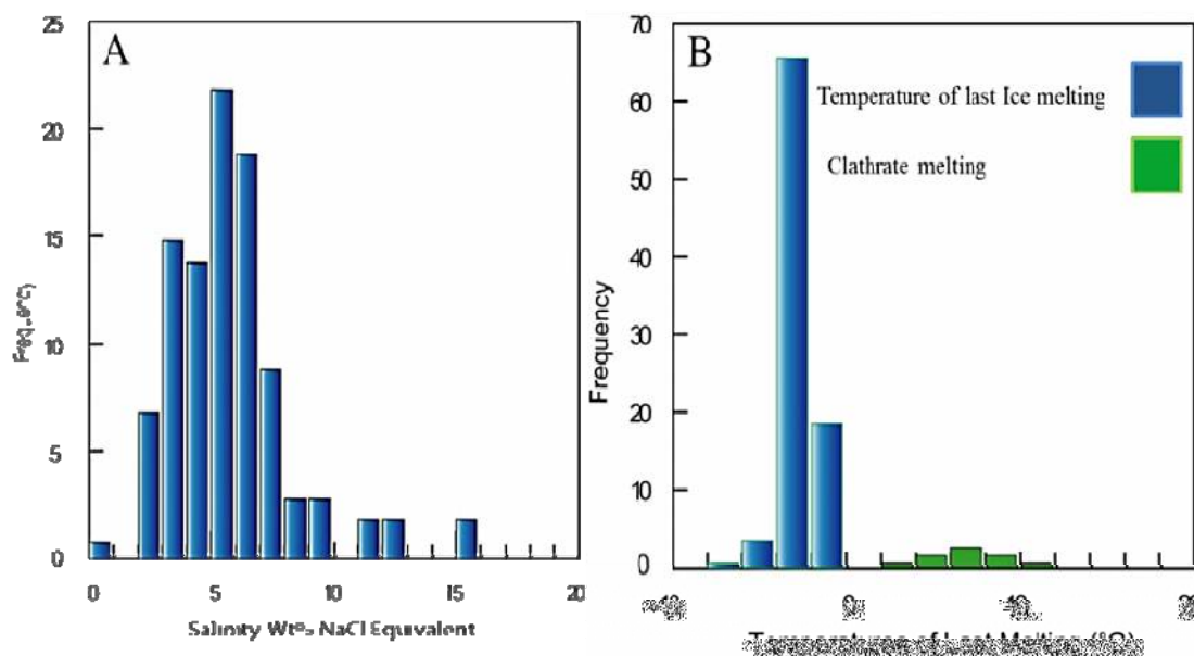
شکل ۱۱. A. نمودار فراوانی شوری سیالات درگیر در کانی کوارتز و B. نمودار فراوانی دمای نهایی ذوب یخ و کلاتریت
