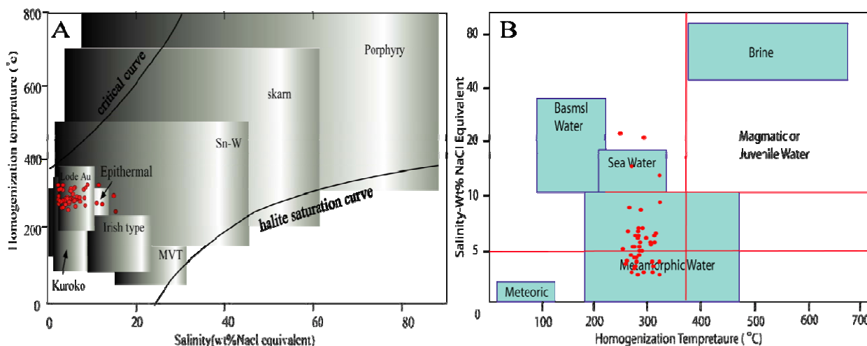
شکل ۱۳. نمودار تعیین نوع کانه‌زایی با استفاده از شوری و دمای همگن‌شدن (Wilkinson, 2001) و B: نمودار تعیین منشأ سیال گرمایی (Kesler, 2005)
