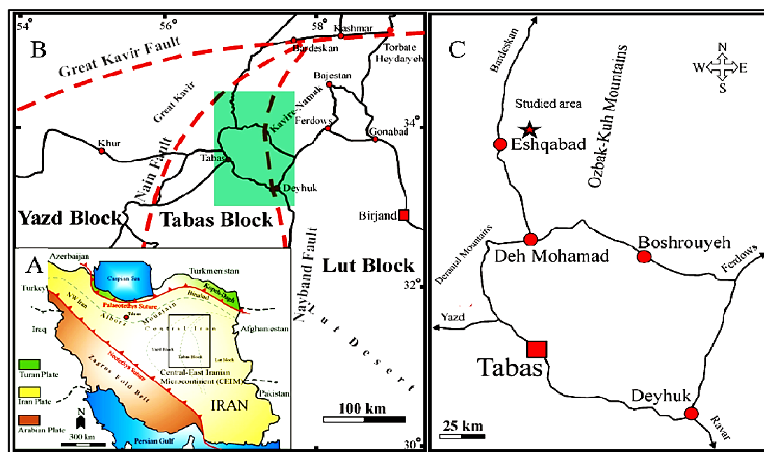
شکل ۱. موقعیت مکانی منطقه دهنو-عبید، A: موقعیت منطقه بر روی نقشه ایران به همراه خط درزه‌های مهم و ساختارهای زمین‌ساختی ورقه ایران برگرفته از ویلمسن و همکاران (Wilmsen et al., 2009)، B: نمایی نزدیکتر از چهارگوش، قسمت شرقی ایران مرکزی و بلوک طبس برگرفته از ویلمسن و همکاران (Wilmsen et al., 2010) و C: موقعیت منطقه مورد بررسی در شمال شرقی شهر عشق‌آباد مشخص شده است برگرفته از زندهمقدم و همکاران (Zand Moghadam et al., 2014) با اندکی تغییرات
