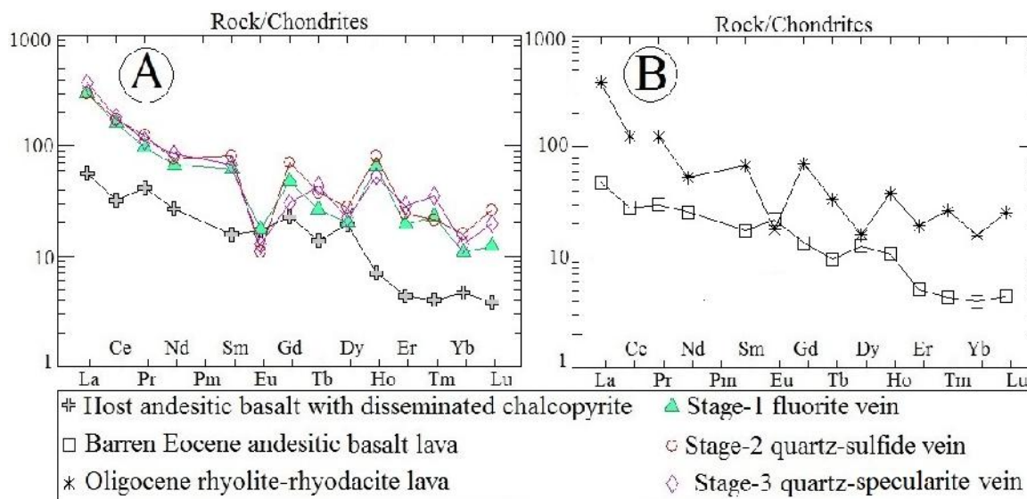
شکل ۱۲. A: الگوی عناصر نادر خاکی به‌هنگار شده نسبت به کندریت (Nakamura, 1974) برای بخش‌های کانه‌دار در رخداد معدنی مس آق کند و B: الگوی عناصر نادر خاکی به‌هنگار شده نسبت به کندریت (Nakamura, 1974) برای گدازه‌های بازالت آندزیتی سالم و بدون کانه‌زایی ائوسن و گدازه‌های ریولیتی-ریوداسیتی الیگوسن در رخداد معدنی مس آق کند
