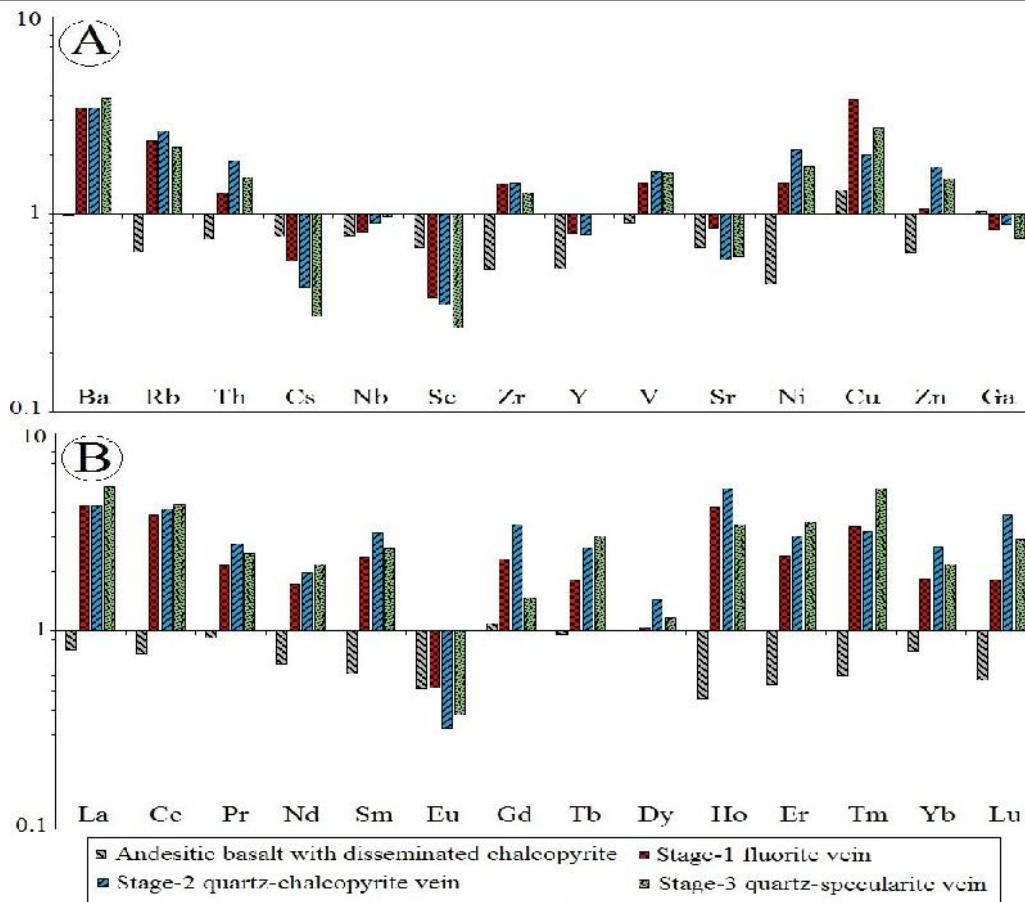
شکل ۱۳. A: نمودار عناصر کمیاب برای بخشهای کانه‌دار در رخداد معدنی مس آق‌کند که نسبت به گدازه بازالت آندزیتی سالم و بدون کانه‌زایی ائوسن (نمونه AQ-14، جدول ۱) به‌هنگار شده‌اند و B: نمودار عناصر نادر خاکی برای بخشهای کانه‌دار در رخداد معدنی مس آق‌کند که نسبت به گدازه بازالت آندزیتی سالم و بدون کانه‌زایی ائوسن (نمونه AQ-14، جدول ۱) به‌هنگار شده‌اند.
