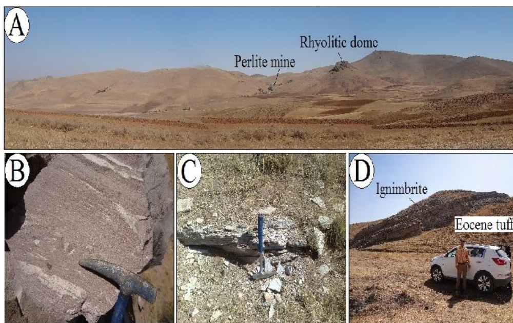
شکل ۲. A: دورنمایی از واحدهای آتشفشانی در منطقه آق‌کند (دید به سمت شمال). در بخش مرکزی تصویر، گنبد ریولیتی-ریوداسیتی و معدن پرلیت دیده می‌شود، B: نمایی نزدیک از لایه‌بندی موجود در گدازه‌های ریولیتی-ریوداسیتی، C: توف‌های ریولیتی-ریوداسیتی الیگوسن و D: لایه‌های ایگنیمبریتی در منطقه آق‌کند (دید به سمت شمال‌خاوری)
