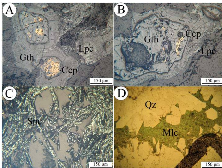
شکل ۹. تصویرهای میکروسکوپی (A تا C در نور بازتابی؛ D در نور عبوری پلاریزه) از مواد معدنی در رخداد معدنی مس آق کند. A و B: بلورهای بی‌شکل کالکوپیریت که توسط کانیهای برون‌زاد گوتیت و لپیدوکروسیت جانشین شده‌اند، C: بلورهای تیغه‌ای اسپکیولاریت و D: مالاکیت با بافت پرکننده فضای خالی بلورهای کوارتز. علائم اختصاری کانیها از ویتنی و اونز (Whitney and Evans, 2010) اقتباس شده است. (Ccp= کالکوپیریت، Gth= گوتیت، Lpc= لپیدوکروسیت، Mlc= مالاکیت، Qz= کوارتز، Spc= اسپکیولاریت)
