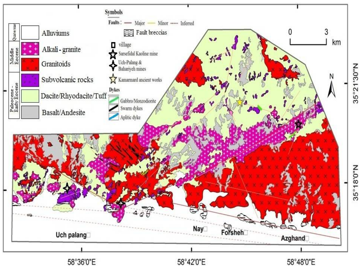
شکل ۲. نقشه زمین‌شناسی منطقه مورد بررسی کاشمر
