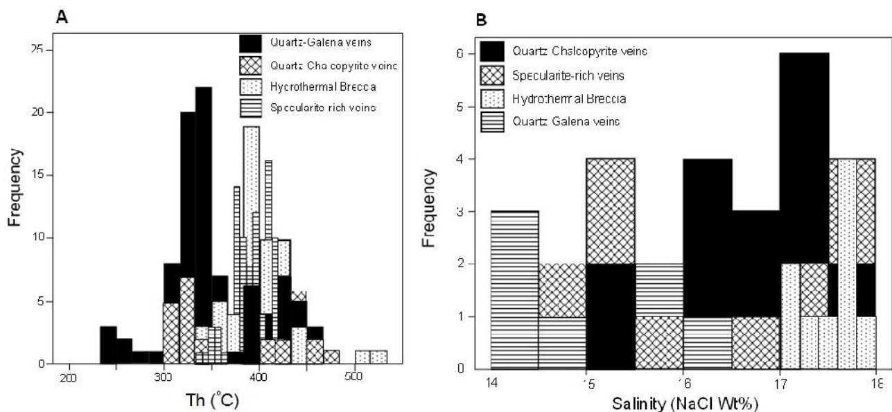
شکل ۱۳. A: هیستوگرام دماهای همگن‌سازی سیالات درگیر انواع رگه‌های کوارتز کانه‌دار کاشمر و B: هیستوگرام شوری سیالات درگیر انواع رگه‌های کوارتز کانه‌دار کاشمر
