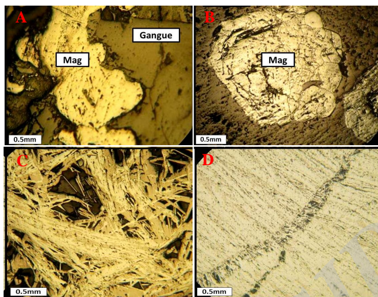
شکل 19. A: حضور مگنتیت (Mag) به صورت بی‌شکل در واحدهای میزبان کانی‌زایی (نور انعکاسی با بزرگ‌نمایی 100X)، B: وجود مگنتیت شکل‌دار در برش سیلیسی شده (نور انعکاسی با بزرگ‌نمایی 50X)، C و D: تأثیر فرآیندهای Mushketovization بر هماتیت و تبدیل آن به مگنتیت (نور انعکاسی با بزرگ‌نمایی 100X، (Whitney and Evans, 2010)
