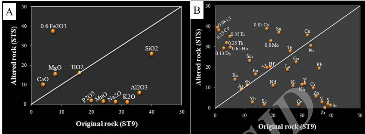
شکل 16. خط هم‌غلظت رسم‌شده برای نمونه STS. A: عناصر اصلی و B: عناصر فرعی
