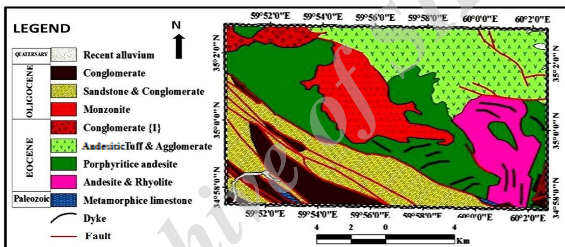
شکل 2. نقشه زمین‌شناسی منطقه رشتخوار (اصلاح شده از نقشه‌های 1:100000 رشتخوار، خواف، دولت‌آباد و کاریزنو (Ancelin et al., 1983) Fig. 2. Geological map of Rhostkhar area (Modified from Roshtkhar, Khaf, Dolatabad and Karizno map, 1/100000) (Ancelin et al., 1983).
