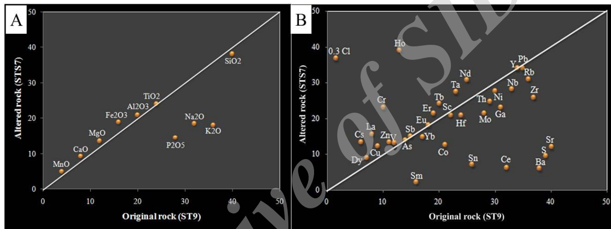
شکل 15. خط هم‌غلظت رسم‌شده برای نمونه STS7. A: عناصر اصلی و B: عناصر فرعی
