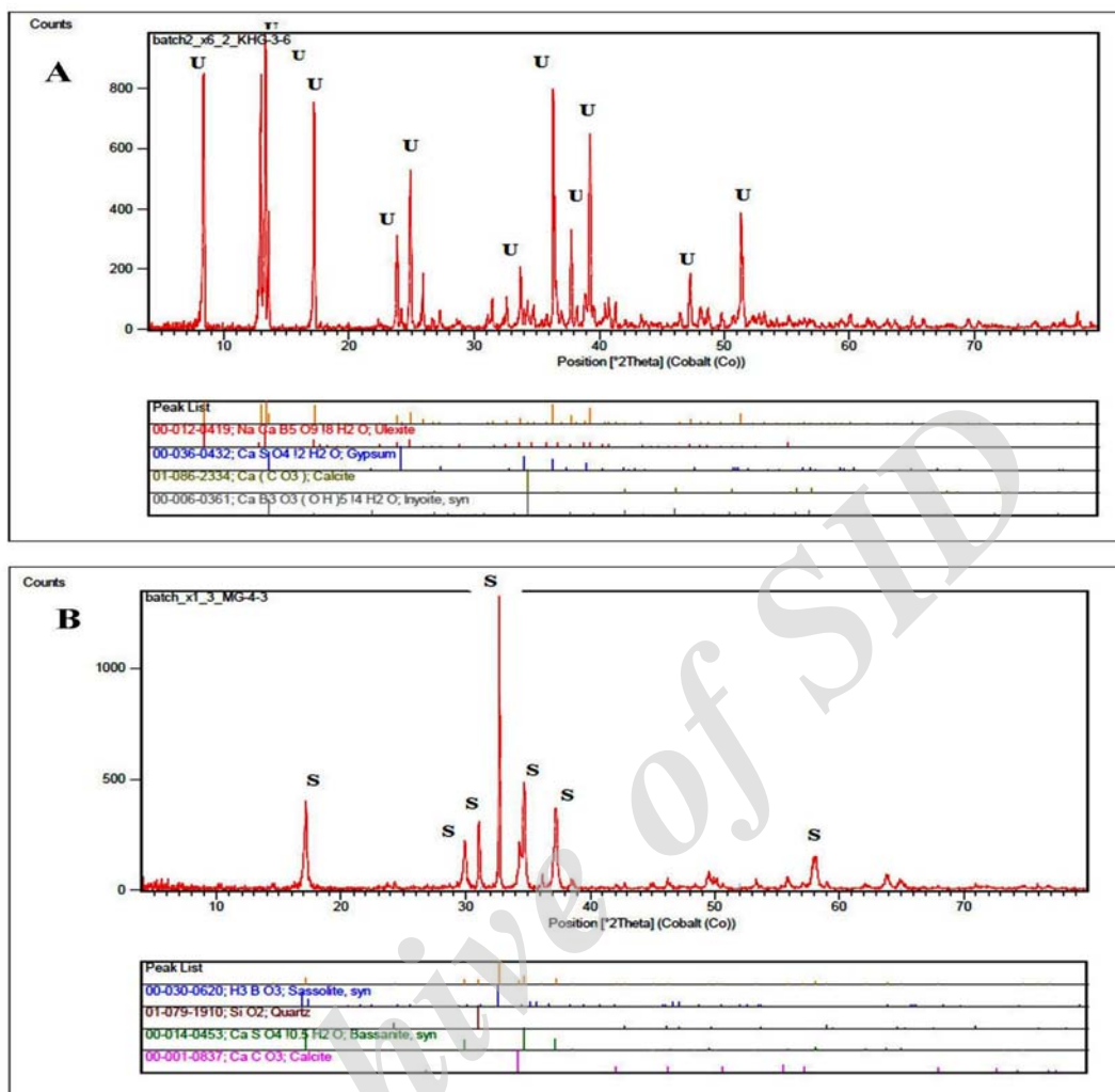
شکل ۷. دو نمونه از پیک‌های XRD مربوط به کانی‌های بوراته مناطق مورد بررسی (پلایای شهربابک): A: پیک مربوط به کانی یولکسیت (U) و B: پیک مربوط به کانی ساسولیت (S)
