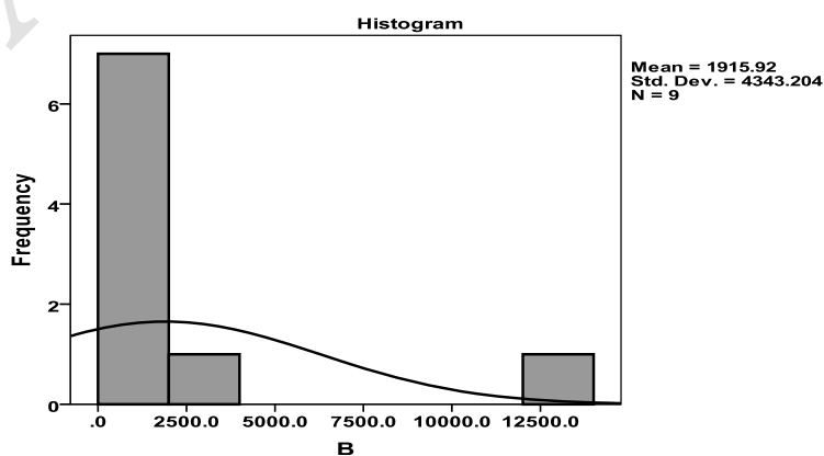
شکل ۸. نمودار فراوانی عنصر بور در مناطق مورد بررسی (پلایای شهربابک)
