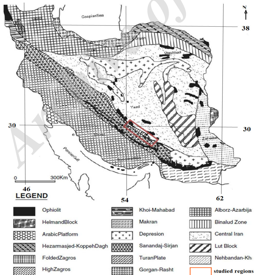
شکل ۱. تقسیم‌بندی واحدهای ساختمانی- رسوبی ایران (Nabavi, 1976) و مناطق مورد بررسی (پلایای شهربابک)
