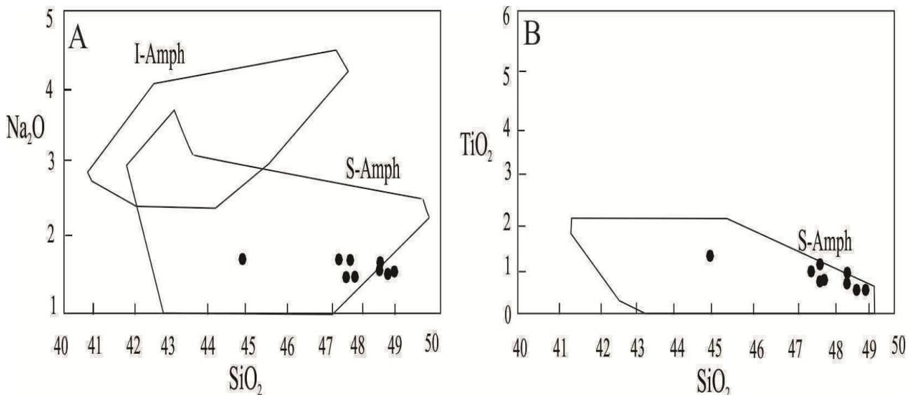
شکل ۸. A: موقعیت آمفیبول‌ها گرانودیوریت تویره در نمودار Na 2 O در مقابل SiO 2 ، برگرفته از کالتورتی و همکاران (Coltorti et al., 2007) و B: موقعیت آمفیبول‌ها گرانودیوریت تویره در نمودار TiO 2 در مقابل SiO 2 ، برگرفته از کالتورتی و همکاران (Coltorti et al., 2007)، در هر دو نمودار، نمونه‌ها در محدوده آمفیبول‌های فرورانش قرار گرفته‌اند.
