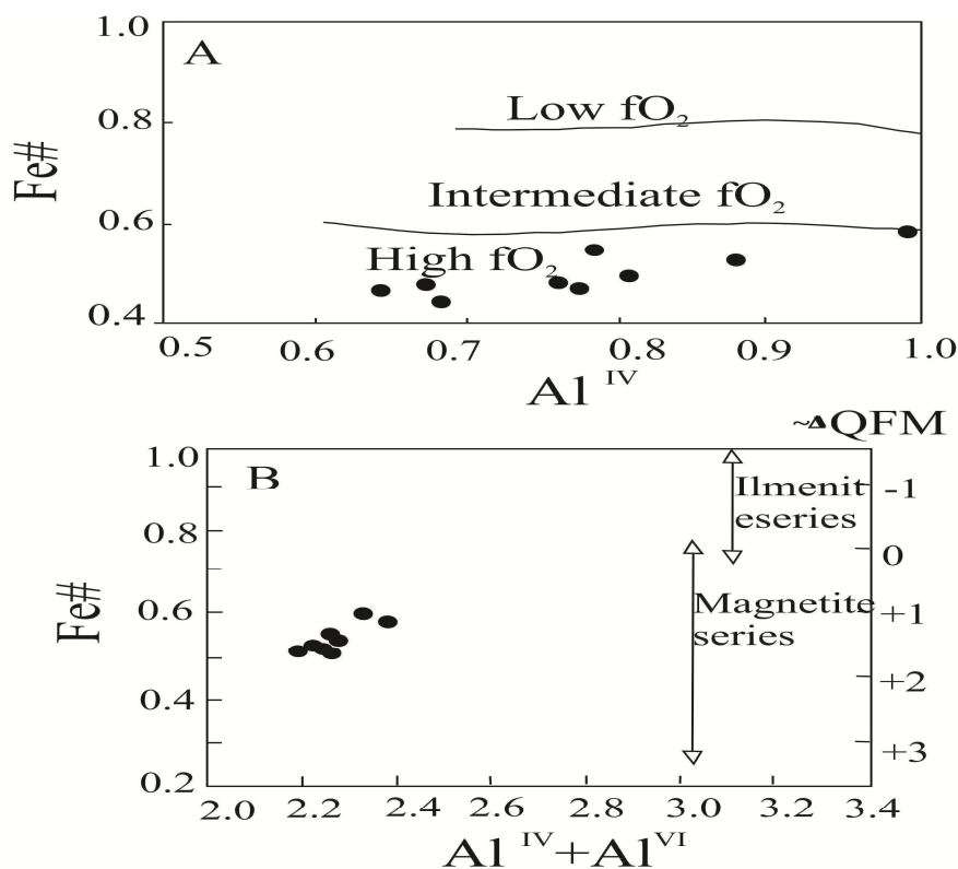
شکل ۱۰. A: نمودار Al^{IV} در برابر Fe# آمفیبول‌های گرانودیوریت تویره، برگرفته از اندرسون و اشمیت (Anderson and Smith, 1995) و B: نمودار Al^{IV}+Al^{VI} در مقابل Fe# بیوتیت‌های گرانودیوریت تویره، برگرفته از اندرسون و همکاران (Anderson et al., 2008) Fig. 10. A: Plot of Al^{IV} versus Fe# for biotite from Toveireh granodiorite (Anderson and Smith, 1995), and B: Binary diagram Al^{IV} + Al^{VI} vs for biotite from Toveireh granodiorite (Anderson et al., 2008)
