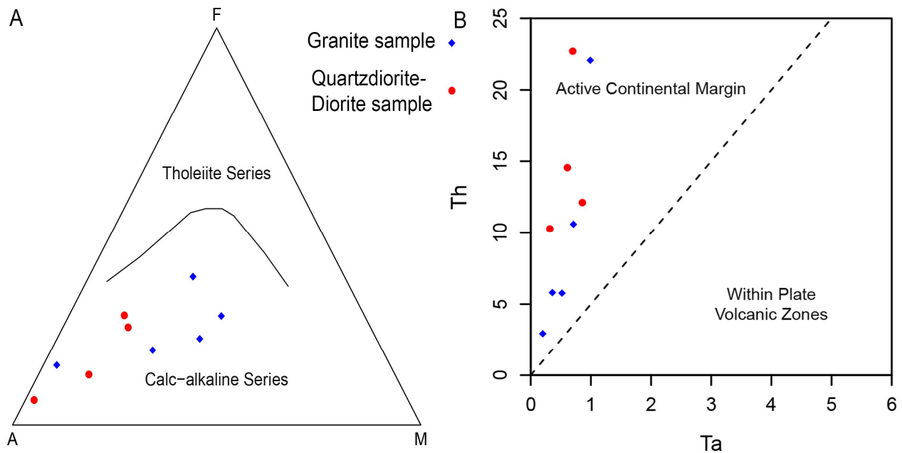
شکل ۱۴. A: ماهیت کالک‌آلکالن سنگ‌های گرانیتی و کوارتز دیوریتی- دیوریتی در محدوده کانسار ساغند (Irvine and Baragar, 1971) و B: موقعیت کمان حاشیه فعال فارهای سنگ‌های گرانیتی و کوارتز دیوریتی- دیوریتی محدوده کانسار ساغند (Schandl and Gorton, 2002)
