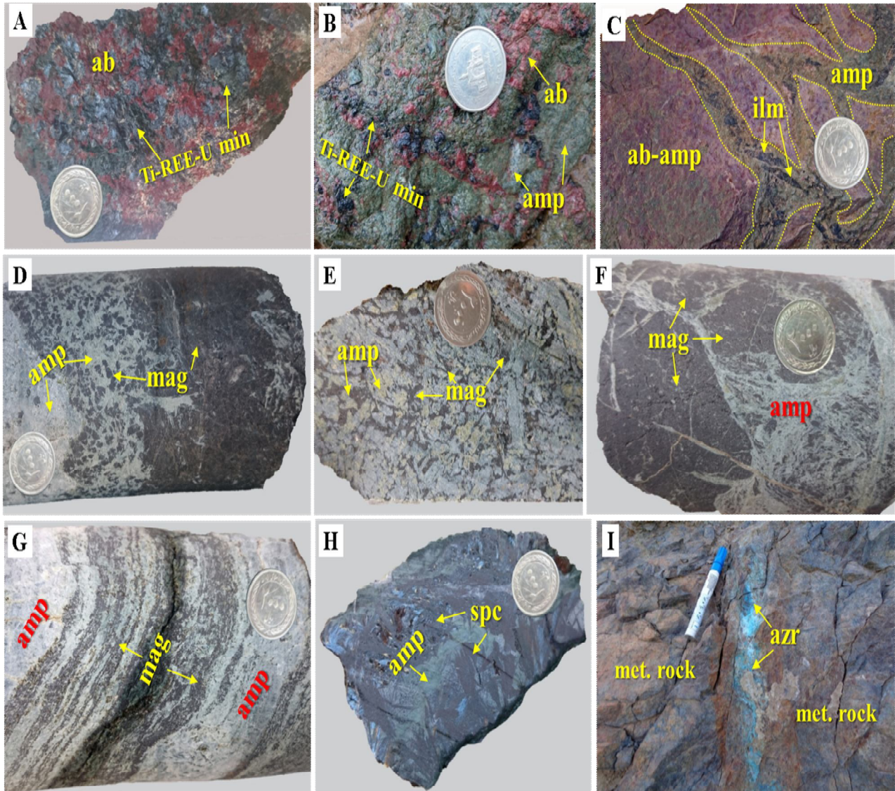
شکل ۶. A: نهشت کانه‌های Ti-REE-U در آلبیت‌های آنومالی پنج ساغند، B: کانی‌سازی افشان Ti-REE-U در دگرنهاد آمفیبولی-آلبیتی، C: رگه‌چه‌های آمفیبول حاوی ایلمنیت که آلبیت-آمفیبول‌های دگرنهادی را قطع کرده‌اند، D: نهشت مگنتیت توده‌ای و افشان در دگرنهاد آمفیبولی، E: مگنتیت فضای بین کانی‌های آمفیبول را پر کرده است، F: برشی شدن مگنتیت‌ها، G: نهشت نوارهای متناوب مگنتیت و آمفیبول، H: اسپکیولاریت‌های ورقه‌ای-رشته‌ای شکل در زمینه دگرنهاد آمفیبولی و I: دگرسانی سوپرژن رگه‌چه سولفیدی مس و تشکیل آزریت در داخل سنگ دگرنهادی. تمام آمفیبول‌ها از گروه اکتینولیت-ترمولیت هستند. ab: آلبیت، amp: آمفیبول، ilm: ایلمنیت، mag: مگنتیت، spc: اسپکیولاریت، آزریت و met.rock: سنگ دگرنهادی، Ti-REE-U min: کانه‌های تیتانیوم، عناصر نادر خاکی و اورانیوم. علائم اختصاری کانی‌ها بر اساس ویتنی و اوانز (Whitney and Evans, 2010)
