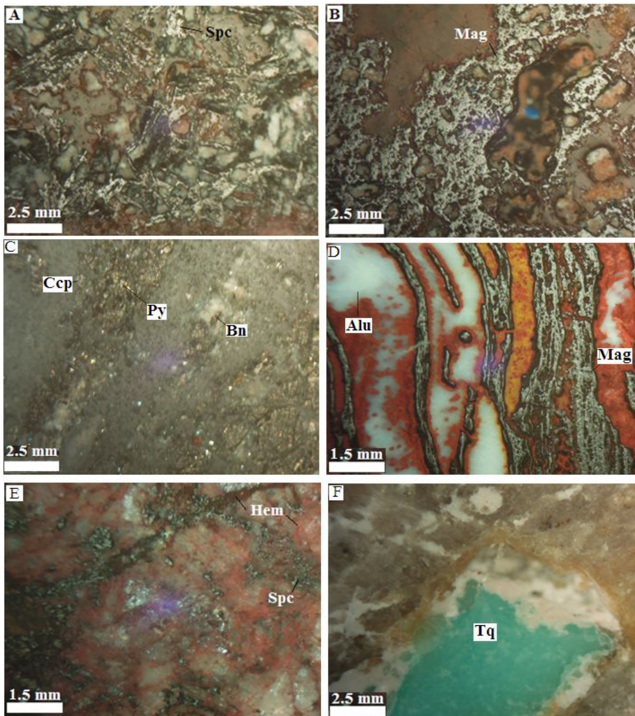
شکل ۷. تصاویر برخی از کانی‌های موجود در ماده معدنی در معدن فیروزه، A: رگه‌چه‌های اسپیکولاریت، B: رگه‌چه مگنتیت در زمینه‌ای برشی، C: دانه‌های پراکنده پیریت، کالکوپیریت و بورنیت، D: رگه‌چه آلونیتی، E: رگه‌چه اسپیکولاریت-هماتیت و F: فیروزه با بافت کلوئیدی. Spc: اسپیکولاریت، Mag: مگنتیت، Ccp: کالکوپیریت، Py: پیریت، Bn: بورنیت، Alu: آلونیت، Hem: هماتیت، Tq: فیروزه. علایم اختصاری بر اساس ویتنی و اوانز (Whitney and Evans, 2010)
