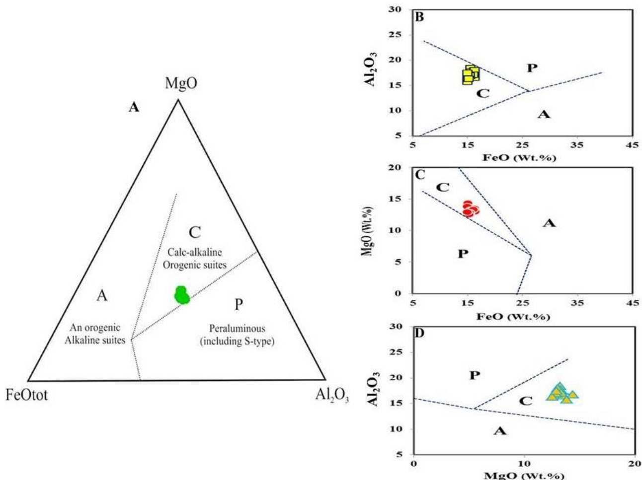
شکل ۸. تطابق بیوتیت‌های ماگمایی چاه فیروزه بر نمودارهای طبقه‌بندی ماگمایی (Abdel-Rahman, 1994). A: نمودار سه‌تایی MgO-FeO-Al 2 O 3 ; B: نمودار دوتایی FeO tot vs. Al 2 O 3 ؛ C: نمودار دوتایی FeO (wt.%) در مقابل Al 2 O 3 (wt.%)؛ D: نمودار دوتایی MgO (wt.%) در مقابل FeO (wt.%)
