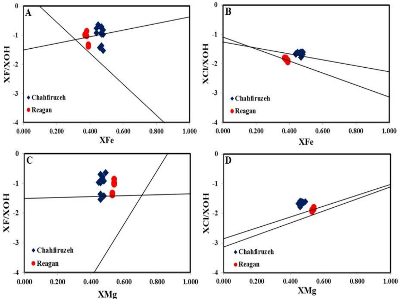
شکل ۱۲. A: \log(XF/XOH) در مقابل \log(XCl/XOH) در مقابل XFe ; B: \log(XCl/XOH) در مقابل XFe ; C: \log(XF/XOH) در مقابل XMg ; D: \log(XCl/XOH) در مقابل XMg برای بیوتیت ماگمایی کانسارهای چاه فیروزه (پورفیری برخوردی) و ریگان (پورفیری پیش از برخورد)
