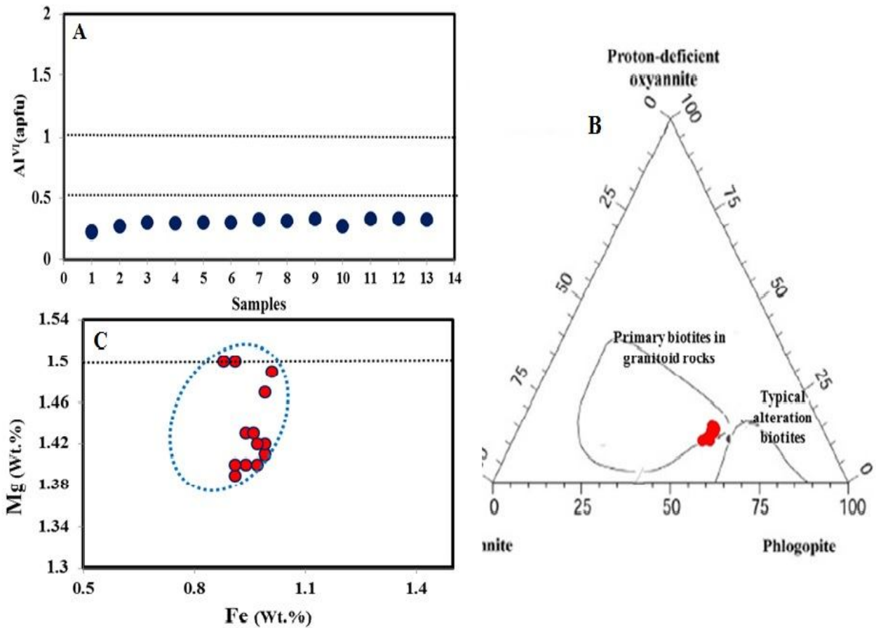
شکل ۷. ترکیب شیمیایی بیوتیت‌های پورفیری چاه فیروزه در A: نمودار فراوانی Al^{IV} (Nachit et al, 2005)، B: نمودار تفکیک مولی بین Al^{IV} و Mg/Fe (Beane, 1974) و C: نسبت Mg/Fe (Beane, 1974)
