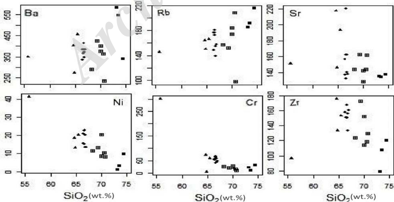
شکل ۶. نمودارهای هارکر عناصر کمیاب (برحسب ppm) در برابر سیلیس در نمونه‌های منطقه کلاه‌قازی. علائم مشابه شکل ۴ هستند.
