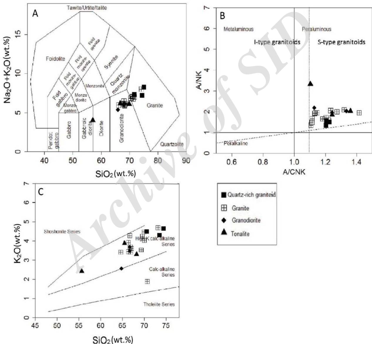
شکل ۴. A: نمودار رده‌بندی ژئوشیمیایی نمونه‌های کلاه‌قازی (Middlemost, 1985). B: نمودار تعیین شاخص اشباع از آلومین (Shand, 1951). C: نمودار تعیین دسته ماگمایی (Peccerillo and Taylor, 1976) با استفاده از مقادیر اکسیدهای عناصر اصلی
