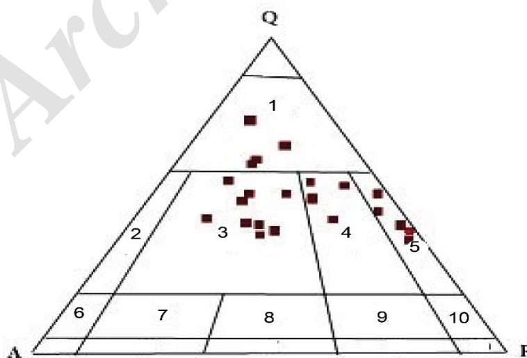
شکل ۲. رده‌بندی مودال سنگ‌های آذرین کلاه قاضی (Streckeisen, 1976): ۱: گرانیتوئید غنی از کوارتز، ۲: گرانیت آلکالن، ۳: گرانیت، ۴: گرانودیوریت و ۵: تونالیت
