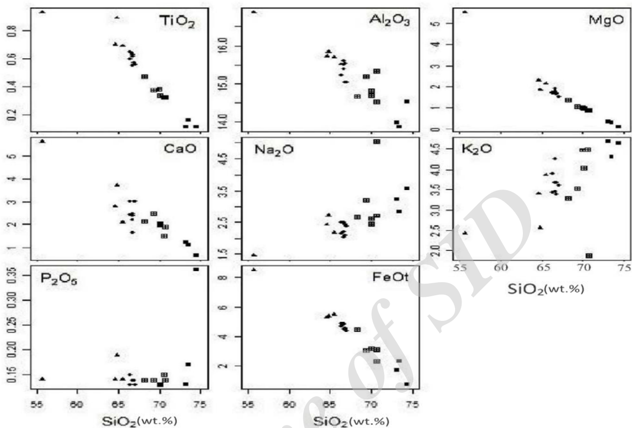
شکل ۵. نمودارهای هارکر عناصر اصلی از نمونه‌های گرانیتوئیدهای کلاه‌قازی. علائم مشابه شکل ۴ هستند.
