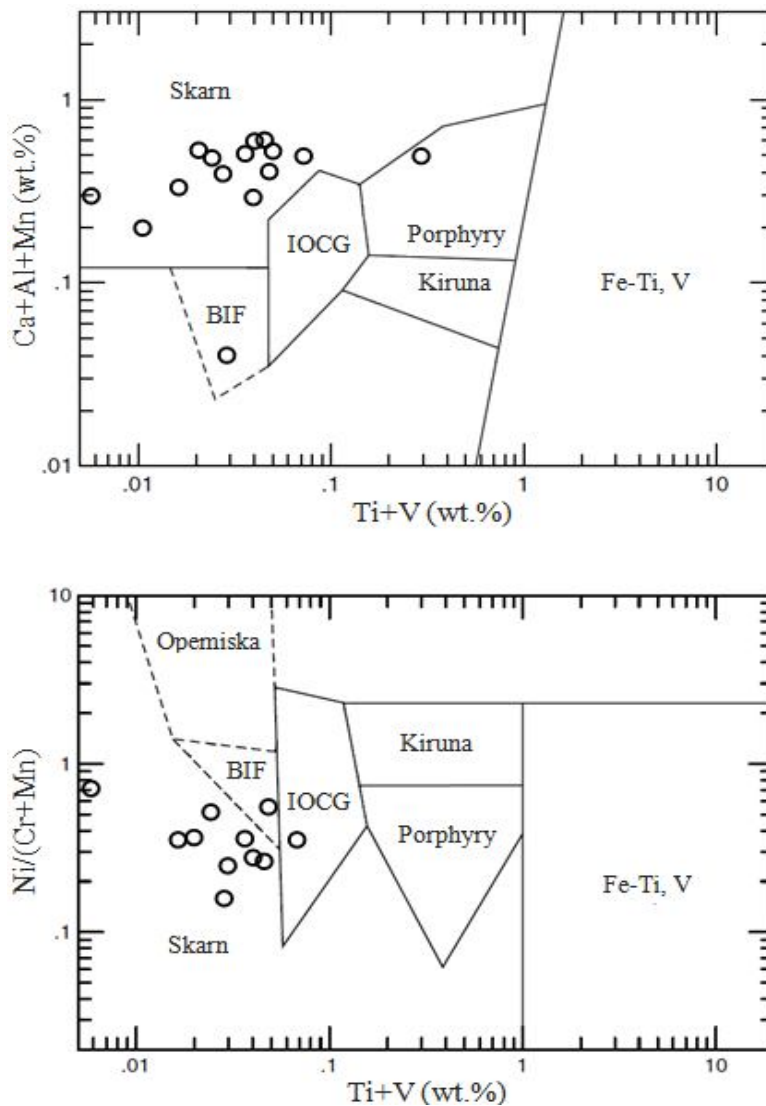
شکل ۱۰. موقعیت نمونه‌های کانی مگنتیت کانسار آهن گوزل‌دره در نمودارهای Ca+Al+Mn در مقابل Ti+V (بالا) و Ni/(Cr+Mn) در مقابل Ti+V (پایین). محدوده‌های مرجع از دوپوئز و بودوین (Dupuis and Beaudoin, 2011)
