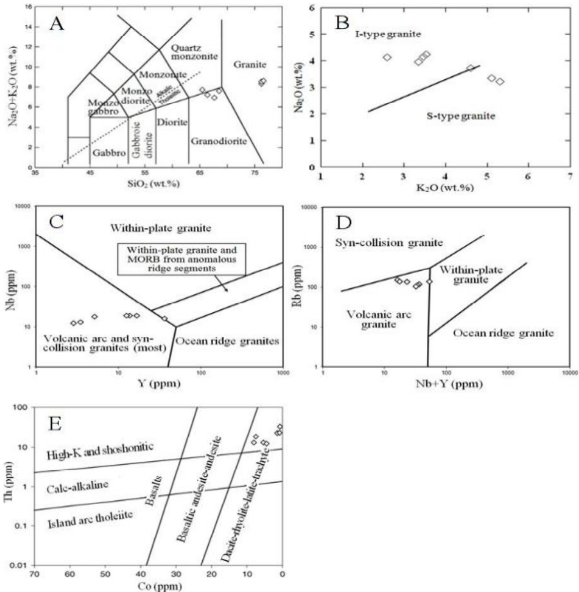
شکل ۵. نام‌گذاری و تعیین نوع توده نفوذی گرانیتوئید گوزل‌دره با استفاده از داده‌های زمین‌شیمیایی. A: نام‌گذاری نمونه‌های توده نفوذی گوزل‌دره با استفاده از نمودار مجموع آلکالی-سیلیس (Middlemost, 1994)، B: تعیین نوع گرانیتوئید گوزل‌دره با استفاده از نمودار \text{Na}_2\text{O}-\text{K}_2\text{O} (Chappell and White, 2001)، C: نمودار متمایزکننده گرانیت‌ها بر اساس Y-Nb (Pearce et al., 1984) برای نمونه‌های گرانیتوئید گوزل‌دره، D: نمودار دو متغیره (Y+Nb)-Rb برای نمونه‌های گرانیتوئید گوزل‌دره (Pearce et al., 1984) و E: نمودار Th-Co برای تفکیک سری‌های تولئیتی، کالک‌آلکان، شوشونیتی و کالک‌آلکان پتاسیم بالا (Hastie et al., 2007). VAG: گرانیت‌های کمان آتشفشانی، syn-COLG: گرانیت‌های هم‌زمان با برخورد، WPG: گرانیت‌های درون‌صفحه‌ای و ORG: گرانیت‌های پشته اقیانوسی
