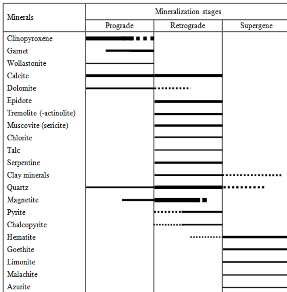
شکل ۹. توالی پاراژنزی کانی‌سازی آهن در منطقه گوزل‌دره
