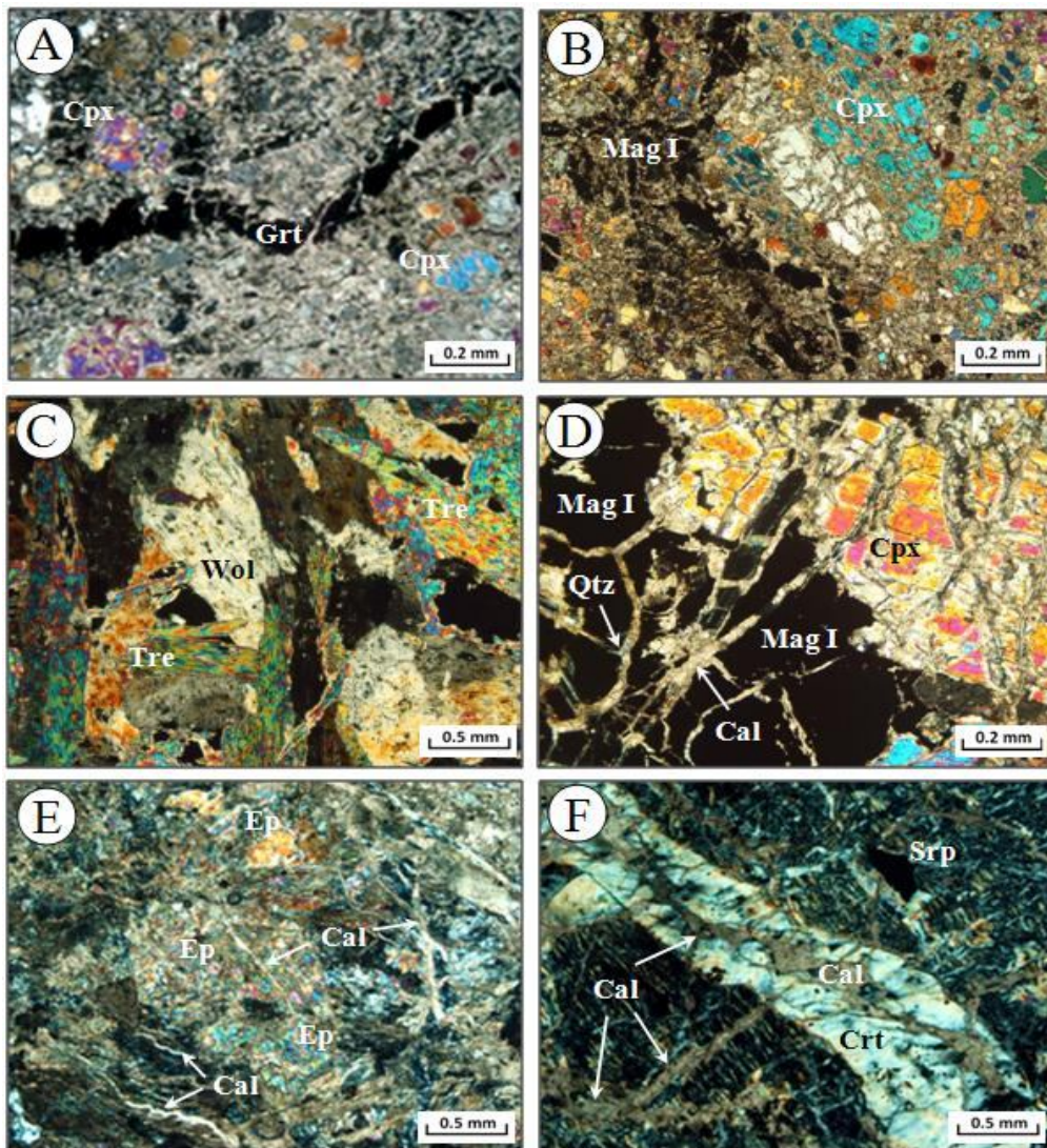
شکل ۷. تصاویر میکروسکوپی کانی‌های سازنده زون اسکارنی کانسار آهن گوزل‌دره. A: تشکیل کلینوپیروکسن پیش‌رونده به همراه رگچه حاوی کانی گارنت پیش‌رونده که آن را قطع می‌کند. هر دو کانی به وسیله رگچه‌های کلسیتی پس‌رونده قطع می‌شوند، B: بلورهای بدوجه کلینوپیروکسن پیش‌رونده به همراه کانی‌سازی اندک مگنتیت پیش‌رونده (Mag I)، C: مجموعه بلورهای کشیده ترمولیت-اکتینولیت پس‌رونده به همراه ولاستونیت پیش‌رونده، D: قطع شدن بلورهای کلینوپیروکسن و مگنتیت پیش‌رونده توسط رگچه‌های تأخیری کلسیت-کوارتز، E: تشکیل اپیدوت در اسکارن پس‌رونده و قطع شدن آن توسط رگچه‌های تأخیری کلسیت و F: تشکیل سرپانتین در اسکارن پس‌رونده و قطع شدن آن توسط رگچه‌های تأخیری کلسیت و کلسیت. Cpx: کلینوپیروکسن، Grt: گارنت، Mag: مگنتیت، Tre: ترمولیت-اکتینولیت، Wol: ولاستونیت، Cal: کلسیت، Qtz: کوارتز، Ep: اپیدوت، Srp: سرپانتین، Crt: کریزوتیل، علائم اختصاری کانی‌ها از ویتنی و اوانز (Whitney and Evans, 2010) اقتباس شده‌اند (تمامی تصاویر در نور پلاریزه عبوری متقاطع گرفته شده‌اند).
