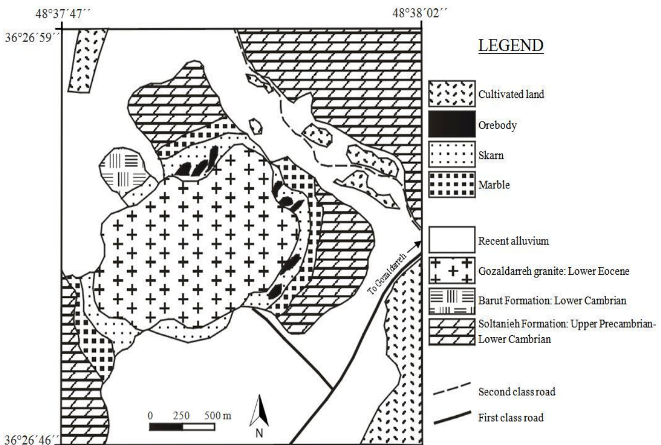
شکل ۳. نقشه زمین‌شناسی کانسار اسکارن آهن گوزل‌دره
