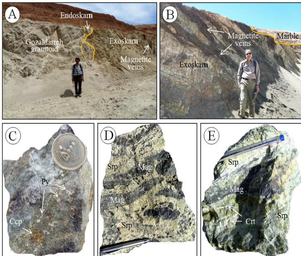
شکل ۶. تصاویر صحرایی و نمونه دستی از کانسار اسکارن آهن گوزل‌دره. A: روابط مکانی توده گرانیتوئید گوزل‌دره با درون‌اسکارن، برون‌اسکارن و کانی‌سازی رگه‌های آهن، B: کانی‌سازی رگه‌های مگنتیت در برون‌اسکارن و تشکیل مرمر در فواصل دورتر، C: تشکیل کانی‌های کالکوپیریت و پیریت در کانسنگ مگنتیت گوزل‌دره، D و E: پیکره‌های نواری مگنتیت در سرپانتین پس‌رونده که توسط رگچه‌های تأخیری کریزوتیل قطع شده است. Ccp: کالکوپیریت، Py: پیریت، Mag: مگنتیت، Srp: سرپانتین، Crt: کریزوتیل، علائم اختصاری کانی‌ها از ویتنی و اوانز (Whitney and Evans, 2010) اقتباس شده‌اند.
