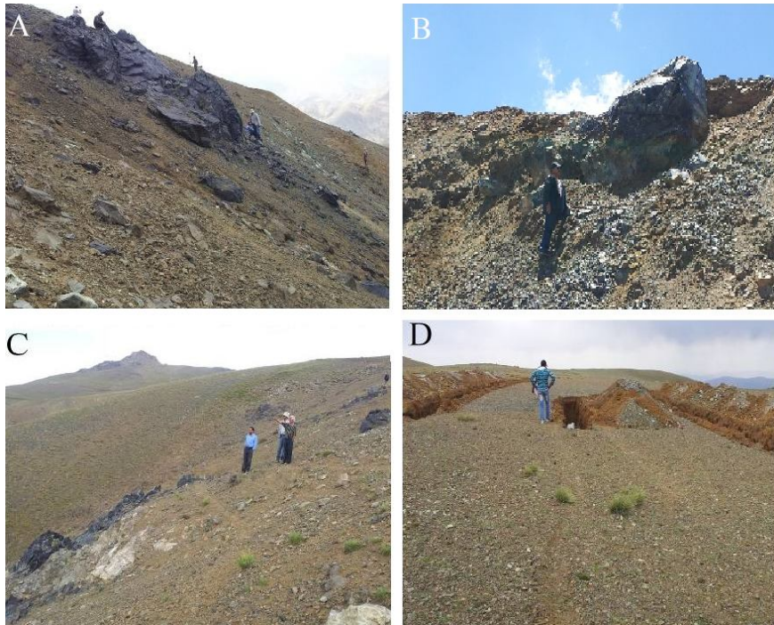
شکل ۶. A و B: رخنمون‌های کرومیتی B1 و C2 صورت لجهای کرومیت در میان سنگ میزبان دیده می‌شوند (به دلیل مقاومت زیادتر آنها در مقابل فرسایش)، C و D: پوشش گیاهی فقیر بر روی مناطق کرومیت‌دار (ناحیه کوچوک)
