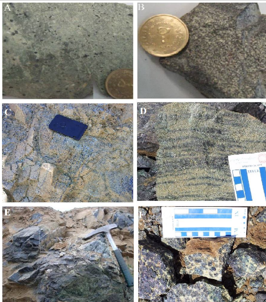
شکل ۵. ساخت و بافت نهشته‌های کرومیتی در ناحیه کوچک. A و B: دانه‌های پراکنده کرومیت در دونیت (پوشش توده کرومیتیتی)، C و D: بافت نواری در بخش حاشیه‌ای و بالایی توده‌های کرومیت، E: بافت متراکم و F: بافت گرهکی (نودولار)
