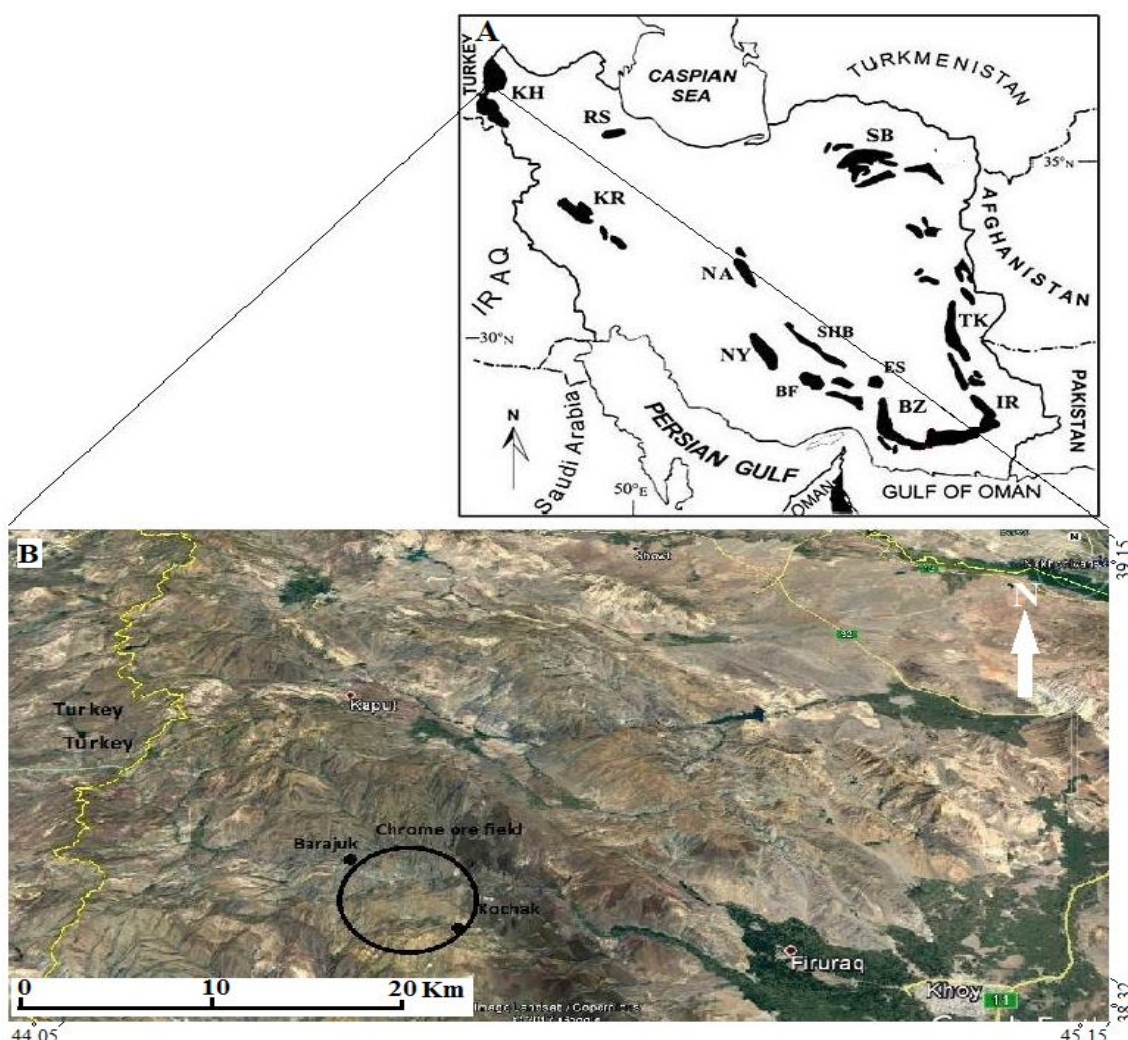
شکل ۱. ۱: پراکندگی افیولیت‌های عمده ایران، نیریز (NY)، اسفندقه (ES)، سبزواری (SB)، نائین (NA)، بافت (BF)، کرمانشاه (KR)، شرق ایران (ایران‌شهر - چهل کوره) (TK-IR) (Ghorbani, 2008) و ۲: موقعیت میدان کروم‌دار کوچوک در افیولیت خوی
