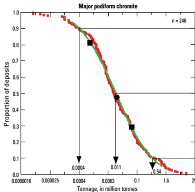
شکل ۷. نمودار عیار-تناژ ذخایر کرومیت انبانی (United States Geological Survey, 2012) و مقادیر بیشینه، میانگین و کمینه ذخایر کرومیتی شناخته‌شده در ناحیه کوچوک
