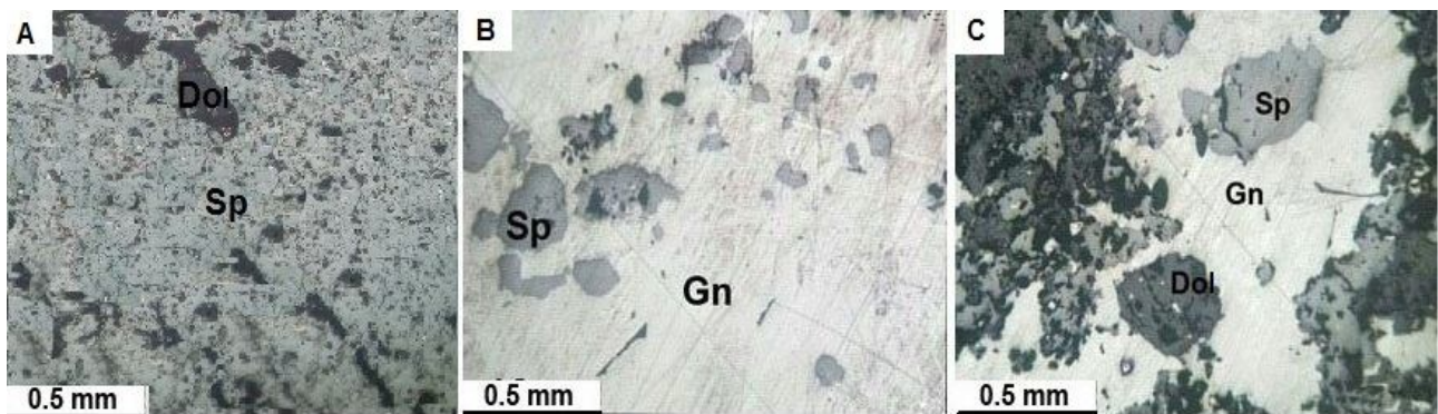
شکل ۴. تصاویر میکروسکوپی از کانه‌های کانسار طرز. A: اسفالریت به‌صورت جانشینی در دولومیت، B: ادخال‌هایی از کانی اسفالریت در گالن و C: ادخال‌هایی از کانی اسفالریت و دولومیت در گالن. علائم اختصاری کانی‌ها از ویتنی و اوانز (Whitney and Evans, 2010) اقتباس شده است (Sp: اسفالریت، Gn: گالن، Dol: دولومیت).
