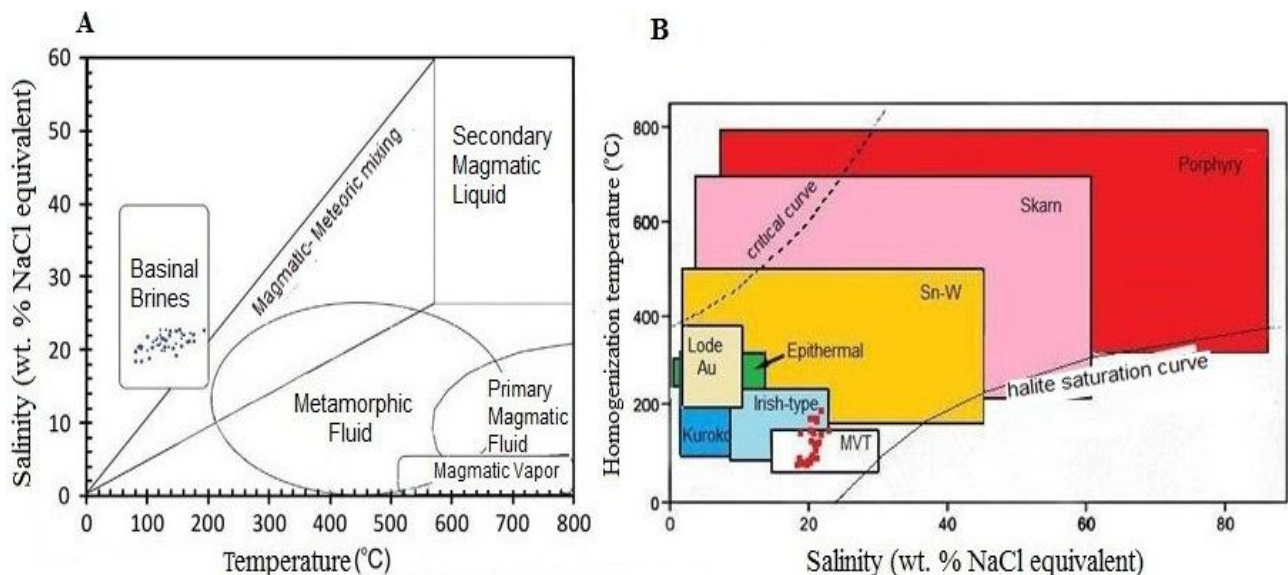
شکل ۱۱. A: نمودار دمای همگن شدن-درجه شوری با تغییرات از بین (Beane, 1983) نشان‌دهنده نوع سیال گرمابی تشکیل‌دهنده کانسار طرز و
