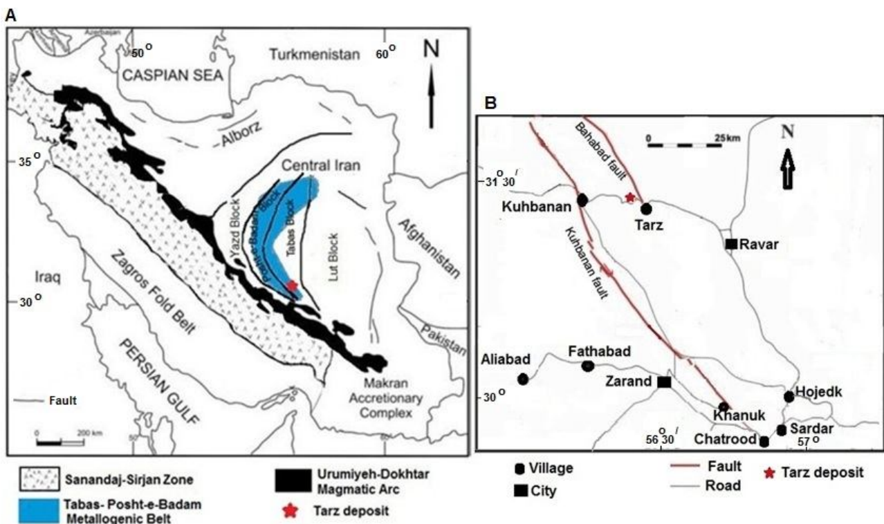
شکل ۱. A: نقشه عمومی ساختاری ایران با تغییرات از اشتوکلین (Stöcklin, 1968) و علوی و همکاران (Alavi et al., 1997) و موقعیت منطقه معدنی طرز در نوار فلززایی طبس-پشت‌بادام و B: نقشه جغرافیایی نشان‌دهنده راه‌های دسترسی به کانسار طرز
