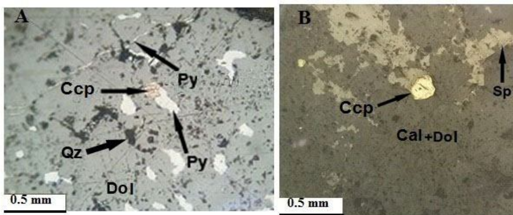
شکل ۵. تصاویر میکروسکوپی نور انعکاسی از کانه‌های کانسار طرز A: پیریت (نسل ۱) و کالکوپیریت جانشین شده در دولستون، رگچه پیریت (نسل ۲) و B: کالکوپیریت و اسفالریت جانشین شده در سنگ کربناتی. علائم اختصاری کانی‌ها از ویتنی و اوانز (Whitney and Evans, 2010) اقتباس شده است (Sp: اسفالریت، Cal: کلسیت، Dol: دولومیت، Ccp: کالکوپیریت، Qz: کوارتز، Py: پیریت).
