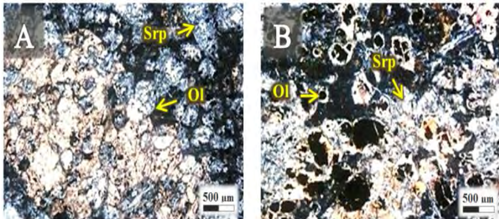
شکل ۳. A: جانشینی سرپانتین به جای الیوین و B: باقی ماندن قالب‌های مدور الیوین با افزایش سرپانتینی شدن (جنوب غرب مشهد). علایم اختصاری از ویتنی و اوانز (Whitney and Evans, 2010) اقتباس شده است (Srp: سرپانتین، Ol: الیوین).
