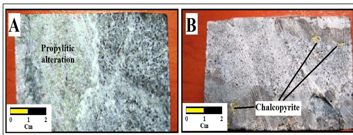
شکل ۳. A: دگرسانی پروپیلیتیک رخ داده در زون اسکارن در مجاورت توده نفوذی در مغزه حفاری در کانسار مزرعه و B: نمای از مغزه حفاری در زون اسکارن مینرالیزه کانسار مزرعه که کانه‌زایی مس (کالکوپیریت) در متن سنگ دیده می‌شود.
