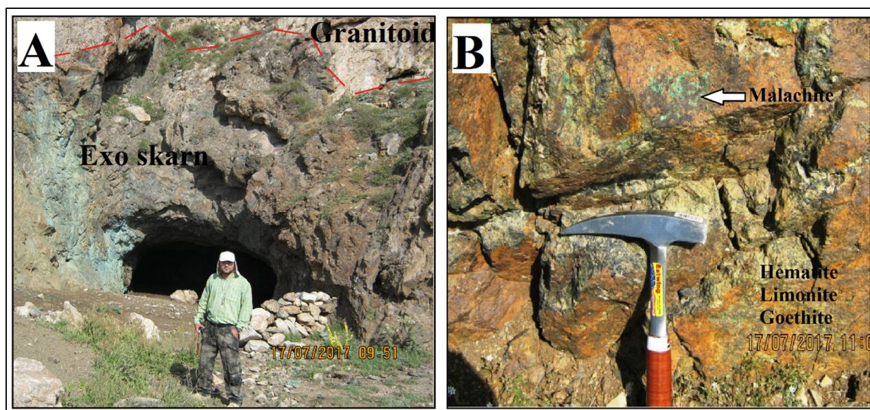
شکل ۲. A: نمای باز از زون اغزواسکارن و کانه‌زایی سطحی (مالاکیت) در همبری با توده گرانیتوئیدی در کانسار مزرعه و B: نمای نزدیک‌تر از زون اغزواسکارن و تشکیل هماتیت، لیمونیت و گوتیت به همراه کانه‌زایی مالاکیت در این زون در کانسار مزرعه
