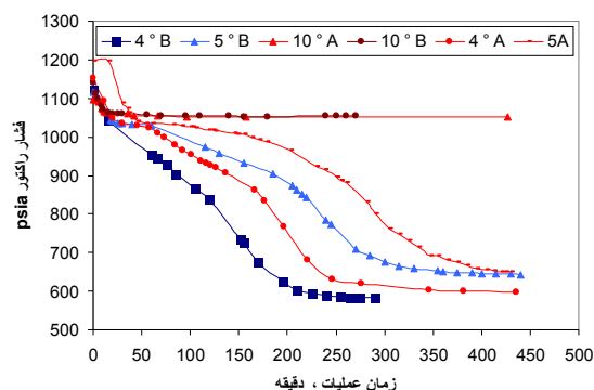
شکل ۷ آزمایش‌های تکراری برای تعیین فشار تعادلی هیدرات در دماهای ۴، ۵ و ۱۰ درجه سلسیوس
