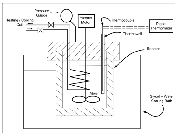
شکل ۳ شمای سامانه به کار گرفته شده برای انجام آزمایش های تشکیل هیدرات گاز متان
