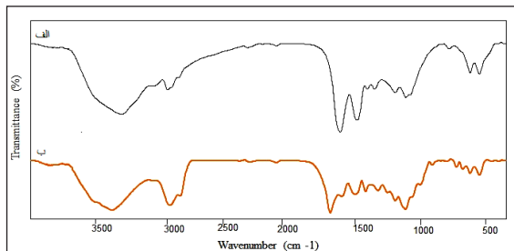
شکل ۱۲ طیف FT-IR انسولین خالص و (ب) نانوکامپوزیت پلی اورتانی مغناطیسی مزدوج با انسولین
