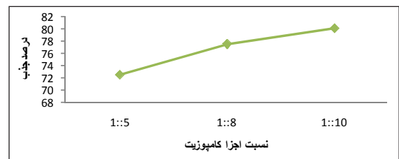
شکل ۸ درصد جذب سرب به وسیله‌ی جاذب هالوسایت نانولوله/گرافن اکسید با تغییرات نسبت جاذب
