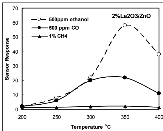
شکل ۴ حساسیت روی اکسید حاوی ۲ درصد لانتانیم اکسید نسبت به گازهای متان، اتانول و CO
