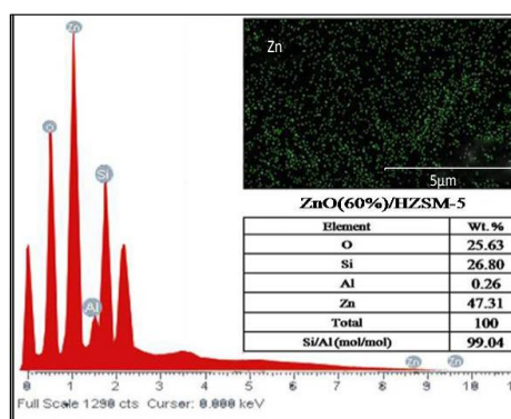
شکل ۳ طیف EDX نانوجندسازه ZnO/HZSM-5
