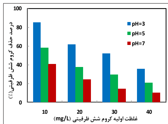
شکل ۶ نمودار تأثیر تغییرات pH بر روی فرایند حذف کروم شش ظرفیتی (زمان برابر ۶۰ دقیقه)
