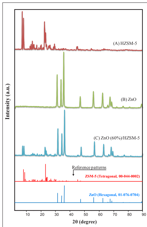
شکل ۱ الگوهای XRD مربوط به (A) زئولیت HZSM-5، (B) نانوذرات ZnO و (C) نانوحندسازه ZnO/HZSM-5
