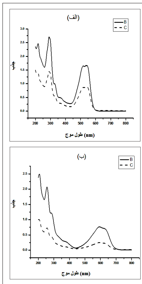
شکل ۵- طیف جذبی UV-vis (الف) محلول رنگزای راکتیو قرمز ۱۹۵ و (ب) محلول رنگزای راکتیو آبی ۱۹ پیش (B) و پس (C) از قرار گرفتن در کنار نانو جاذب گرافن اکسید.
