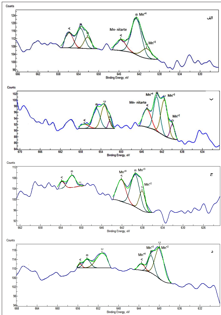
شکل ۷ طیف‌های XPS و انرژی بستگی Mn\ 2p_{1/2} و Mn\ 2p_{3/2} کاتالیست‌های حاوی ۱۲ wt% منگنز اکسید کلسینه شده در دمای (الف) 300^\circ\text{C} ، (ب) 400^\circ\text{C} ، (ج) 500^\circ\text{C} ، د 600^\circ\text{C} به مدت ۳ h
