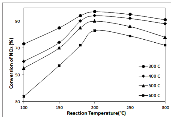
شکل ۲ تأثیر دمای کلسینه شدن بر درصد تبدیل ترکیبات NOx در دماهای متفاوت واکنش
