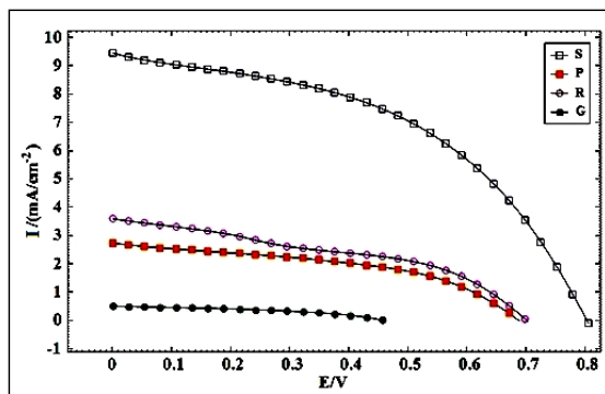
شکل ۲ نمودارهای چگالی جریان - پتانسیل برای سلول‌های خورشیدی رنگدانه‌ای دارای رنگدانه‌های متفاوت (S: رنگدانه استاندارد، P: آب انار، R: چای قرمز و G: چای سبز).
