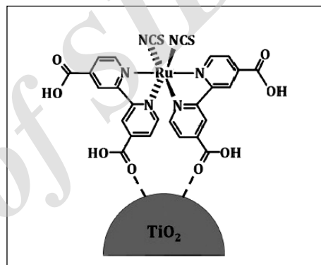
شکل ۱۱ ساختار مولکولی N719 و پیوند بین این مولکول با ذرات TiO_2
