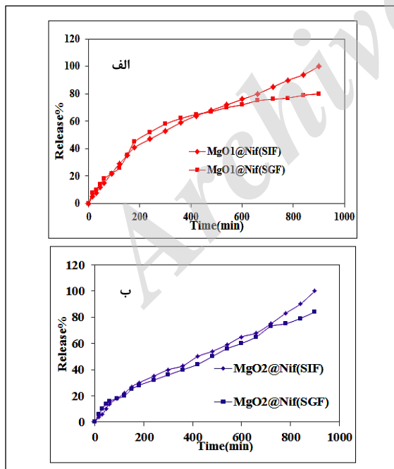
شکل ۵ نمودارهای رهایش نیفدیپین (الف) در محیط معده و روده برای بستر انتخابی MgO1' (ب) در محیط معده و روده برای بستر انتخابی MgO2
