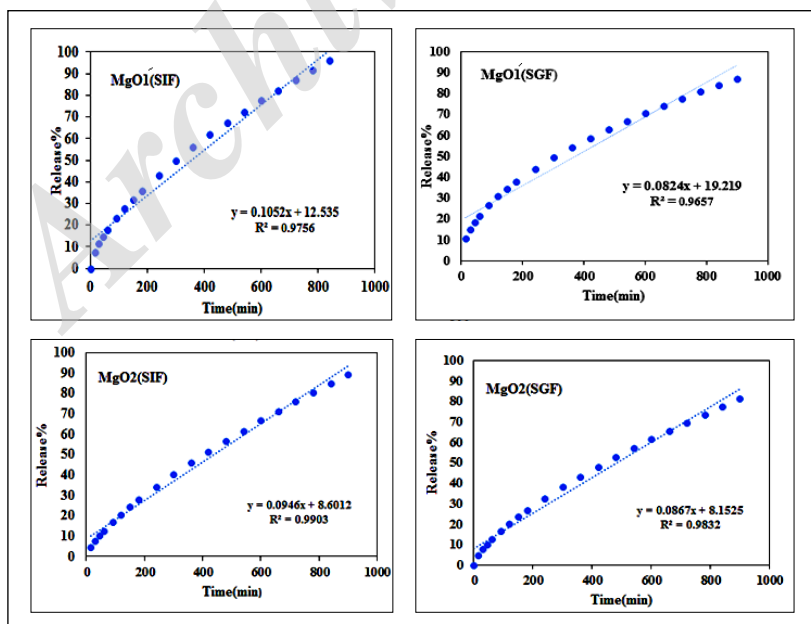
شکل ۶ سینتیک رهایش نیفدیپین از MgO_2 و MgO_1 در محیط معده و روده با استفاده از معادله کورسمایر-پپاس
