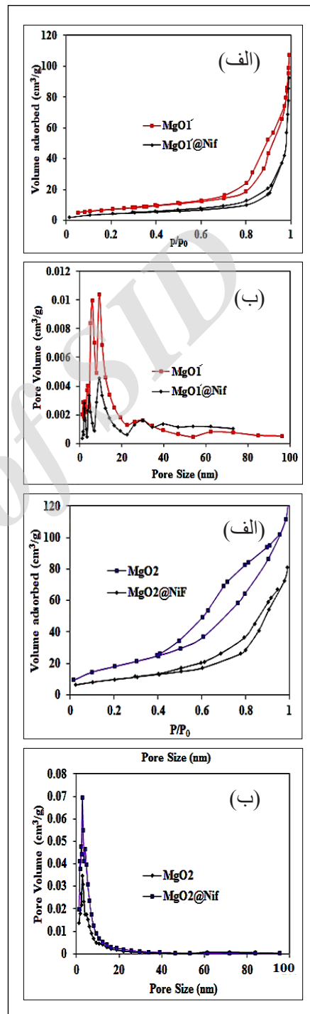
شکل ۱ نمودارهای (الف) هم‌دمای جذب و واجذب نیتروژن مربوط به نمونه‌های MgO_1'@Nif ، MgO_1' و MgO_2@Nif ، MgO_2' و (ب) توزیع اندازه حفره در نمونه‌های MgO_1'@Nif ، MgO_1' و MgO_2@Nif ، MgO_2'
