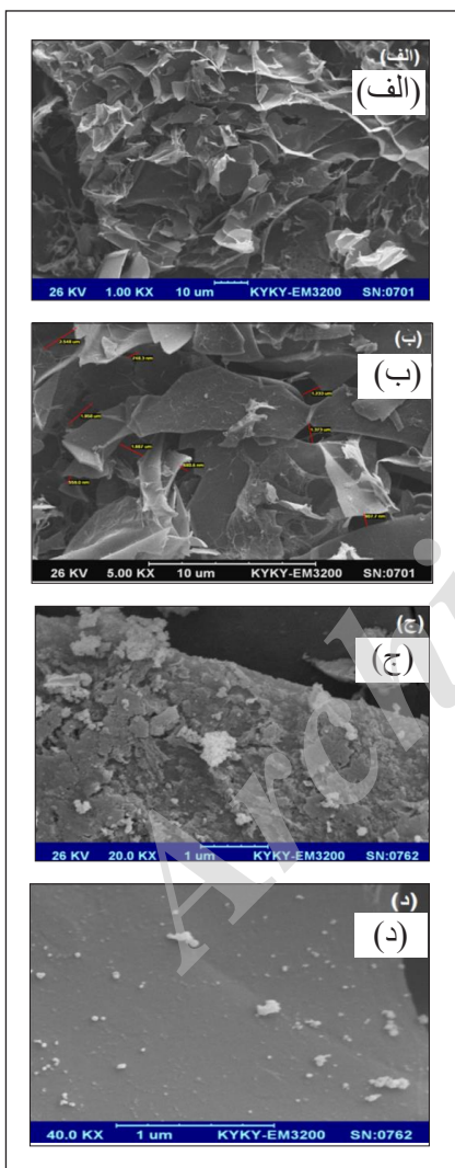
شکل ۵ تصویر میکروسکوپ الکترونی روبشی آب‌ژل با (الف) بزرگنمایی ۱۰۰۰ و (ب) برابر و تصویر میکروسکوپ الکترونی روبشی آب‌ژل‌های نانوجندسازه با بزرگنمایی (ج) ۲۰۰۰۰ و (د) ۴۰۰۰۰ برابر
