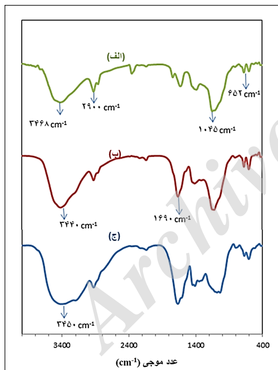
شکل ۷ طیف فرسرخ (الف) صمغ عربی، (ب) آب‌زل، (ج) آب‌زل نانوجندسازه
