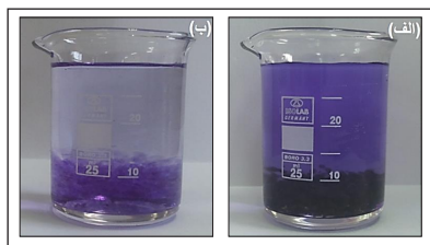
شکل ۴ جذب محلول رنگ بنفش بلوری با آب‌ژل‌های نانوجندساز مغناطیسی، (الف) پیش از جذب رنگ و (ب) پس از جذب رنگ (شرایط جذب: مقدار جاذب ۰/۰۵ گرم غلظت اولیه رنگ ۱۰ میلی‌گرم بر لیتر)
