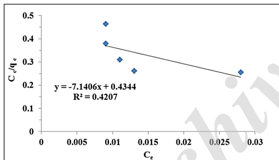
شکل ۱۵ نمودار لانگمویر برای جذب رنگ به‌وسیله آب‌ژل نانوجندسازه (شرایط جذب: مقدار جاذب ۰٫۰۵ گرم، دما ۲۵ درجه سانتی‌گراد)
