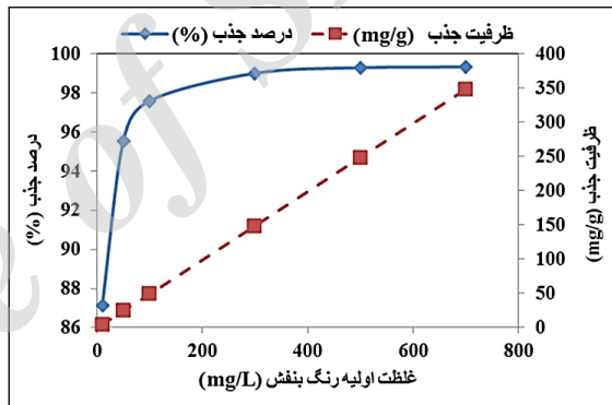
شکل ۱۳ نمودار درصد جذب و ظرفیت جذب و ظرفیت جذب رنگ بنفش بلوری آب‌ژل‌های نانوجندسازه در غلظت‌های بالا (شرایط جذب: مقدار جاذب ۰٫۱ گرم، دما ۲۵ درجه سانتی‌گراد و زمان ۶۰ دقیقه)
