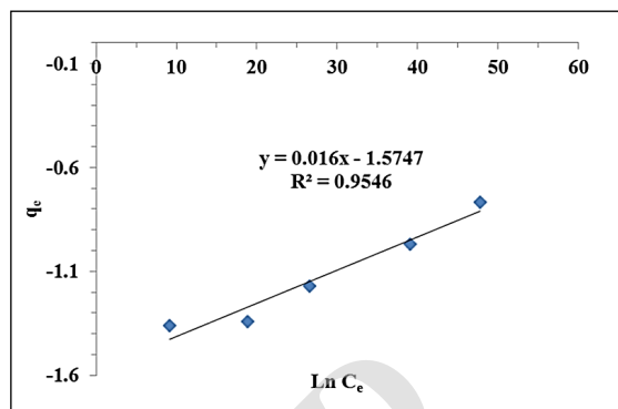
شکل ۱۷ نمودار تمکین برای جذب رنگ به‌وسیله آب‌ژل نانوچندسازه (شرایط جذب: مقدار جاذب ۰٫۰۵ گرم، دما ۲۵ درجه سانتی‌گراد)
