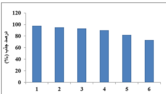
شکل ۱۴ درصد جذب رنگ بنفش بلوری آب‌ژل‌های نانوجندسازه در چرخه‌های متفاوت شرایط جذب (مقدار جاذب ۰٫۰۲ گرم جاذب غلظت اولیه رنگ ۱۰ میلی‌گرم بر لیتر)
