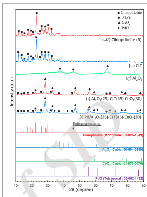
شکل ۶ الگوهای XRD کلینوپتیلولیت طبیعی یا خام (الف)، کلینوپتیلولیت فراوری شده (CLT)، (ب) کلینوپتیلولیت فراوری شده (CLT)، (ج) آلومینا (Clinoptilolite)، (د) \text{Al}_2\text{O}_3(25)\text{-CLT}(45)\text{-CeO}_2(30) و (ه) نانوکاتالیست \text{Pd}/\text{Al}_2\text{O}_3(25)\text{-CLT}(45)\text{-CeO}_2(30) تهیه شده
