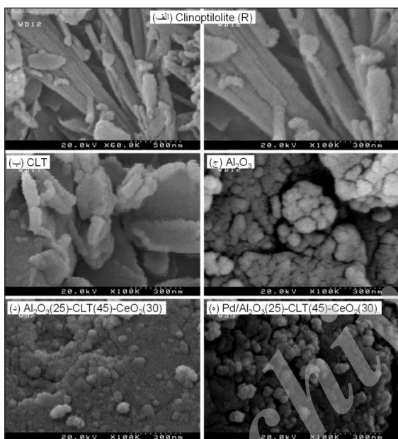
شکل ۷ تصاویر الگوهای FESEM کلینوپتیلولیت طبیعی یا خام (الف)، کلینوپتیلولیت فراوری شده (CLT)، (ج) آلومینا (Clinoptilolite)، (ب) کلینوپتیلولیت فراوری شده (CLT)، (د) \text{Al}_2\text{O}_3(25)\text{-CLT}(45)\text{-CeO}_2(30) و (ه) نانوکاتالیست \text{Pd}/\text{Al}_2\text{O}_3(25)\text{-CLT}(45)\text{-CeO}_2(30) تهیه شده
