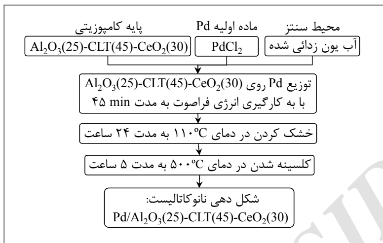
شکل ۳ مراحل سنتز پایه کامپوزیتی \text{Al}_2\text{O}_3\text{-Clinoptilolite-CeO}_2
