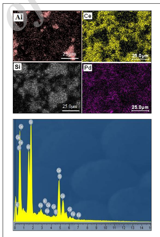
شکل ۹ تجزیه عنصری نانوکاتالیست \text{Pd}/\text{Al}_2\text{O}_3 -Clinoptilolite- \text{CeO}_2 با روش EDS
