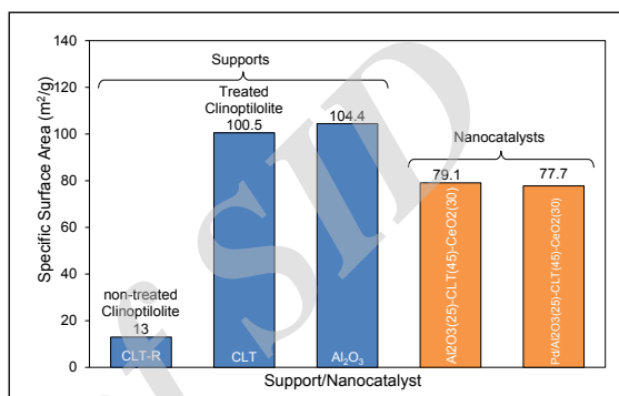
شکل ۱۰ مساحت سطح ویژه پایه و نانوکاتالیست تهیه شده Pd/Al 2 O 3 -Clinoptilolite-CeO 2
