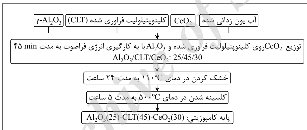
شکل ۴ مراحل سنتز نانوکاتالیست \text{Pd}/\text{Al}_2\text{O}_3\text{-Clinoptilolite-CeO}_2
