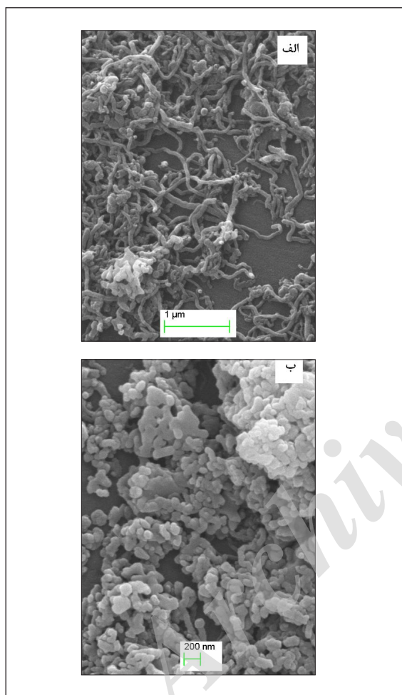
شکل ۲ تصاویر میکروسکوپ الکترونی روبشی سطح الکترودهای GC/MWCNT/Fe 2 O 3 (ب) و GC/MWCNT (الف)
