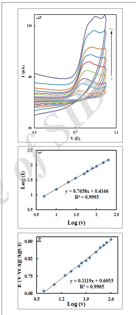
شکل ۴ ولتاموگرام چرخه‌ای 100 \mu\text{M} فنتانیل در سطح الکتروده اصلاح شده در سرعت‌های روبش متفاوت از پایین به بالا ۵ تا 200 \text{ mV s}^{-1} ، (الف) محلول الکترولیت ۰٫۱ مولار فسفات و pH برابر با ۷٫۴، (ب) تغییرات لگاریتم جریان بر حسب لگاریتم سرعت روبش و (ج) تغییرات پتانسیل پیک آندی با لگاریتم سرعت روبش
