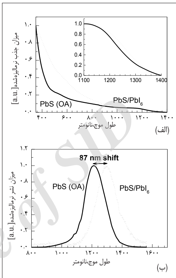
شکل ۷: طیف جذبی نرمالیزه شده (الف) (شکل داخلی نمودار با بزرگنمایی بیشتر در گستره طول موج ۱۱۰۰ تا ۱۴۰۰ nm) و (ب) طیف نشری نرمالیزه شده فیلم‌های سرب سولفید حاوی لیگاند‌های OA و \text{MA}_4\text{PbI}_6
