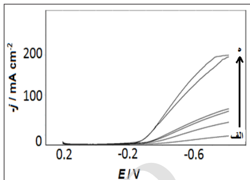
شکل ۷ ولتاگرام‌های روبش خطی فرایند آزادسازی هیدروژن در سطح Pt-CNT/CPE در سولفوریک اسید با غلظت‌های (الف) 0.01، (ب) 0.03، (ج) 0.05، (د) 0.075، (ی) 0.1 و (ه) 0.2 M با سرعت روبش 100 mV s -1
