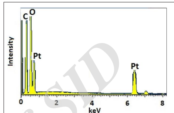
شکل ۳ طیف EDX خمیر کربن اصلاح شده با چندسازه پلاتین بلک و نانولوله‌های کربنی
