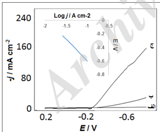
شکل ۵ مقایسه رفتار الکتروکاتالیستی (الف) CPE، (ب) CNT/CPE و (ج) Pt-CNT/CPE، نسبت به فرایند HER در سولفوریک اسید 0.1 M در سرعت روبش 100 mV s -1 ، نمودار تافل برای فرایند HER در سطح Pt-CNT/CPE آزمون سینتیکی واکنش آزادسازی هیدروژن در سطح Pt-CNT/CPE با استفاده از نمودار تافل (شکل ۵) انجام شده
