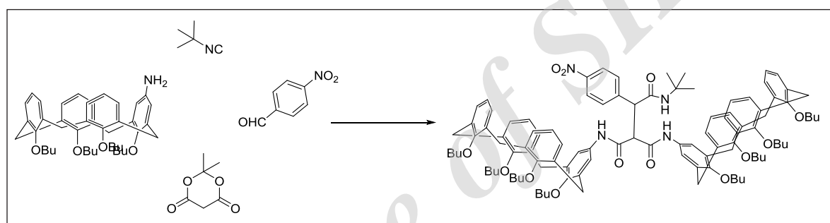
شکل ۱۲. تهیه ترکیب کالیکس [۴] آرن دوپار شده برای شناسایی NADH
