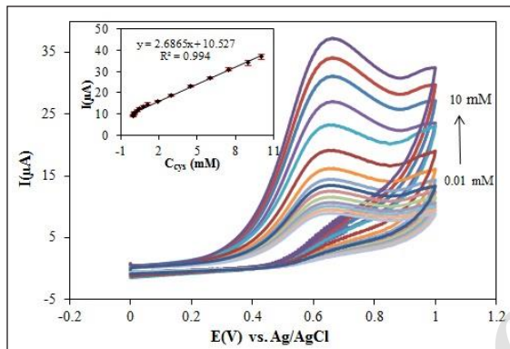
شکل ۹ ولتاموگرام‌های چرخه‌ای ال-سیستین و بافر فسفات در غلظت‌های متفاوت و نمودار تغییرات شدت جریان بر حسب غلظت ال-سیستین
