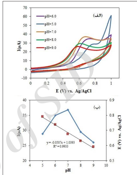
شکل ۷ (الف) ولتاموگرام‌های چرخه‌ای محلول ۱٫۰ میلی مولار ال-سیستین و بافر فسفات در pH های متفاوت در سطح الکتروود GCE/PIN/Ag با سرعت روبش ۱۰۰ میلی ولت بر ثانیه و (ب) نمودار تغییرات شدت جریان و پتانسیل ال-سیستین بر حسب pH
