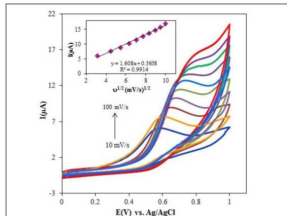
شکل ۸ ولتاموگرام‌های چرخه‌ای محلول ۱٫۰ میلی مولار ال-سیستین و بافر فسفات در سرعت‌های روبش متفاوت به ترتیب از پایین به بالا ۴۰، ۵۰، ۶۰، ۷۰، ۸۰، ۹۰ و ۱۰۰ میلی ولت بر ثانیه و نمودار تغییرات جریان ال-سیستین بر حسب جذر سرعت روبش.
