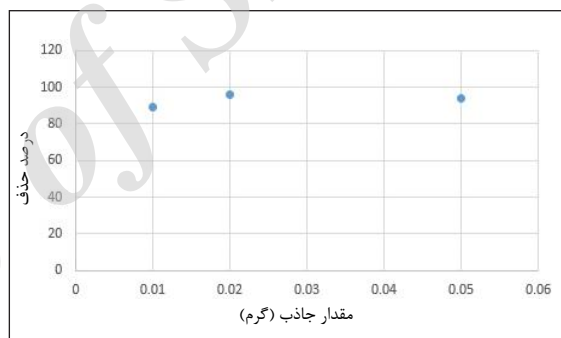
شکل ۸ اثر مقدار جاذب بر درصد حذف آلاینده یون سرب (II) در مجاور نانوجاذب چندسازه سه جزیی گرافن مغناطیسی نایلون ۶
