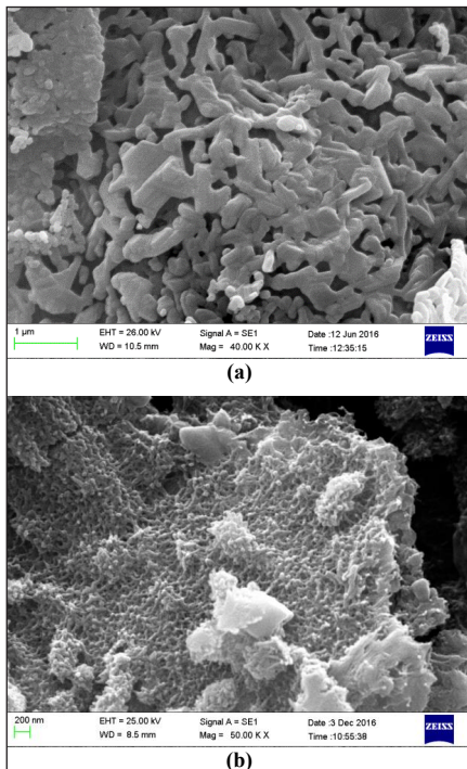
شکل ۳ تصویرهای FESEM نمونه‌های (a) \text{SrFe}_{11.1}(\text{Zn}_{0.5}\text{Co}_{0.5}\text{Zr})_{0.45}\text{O}_{19} و (b) نانوجندسازه پلی‌آنیلین / \text{MWCNTs/SrFe}_{11.1}(\text{Zn}_{0.5}\text{Co}_{0.5}\text{Zr})_{0.45}\text{O}_{19}
