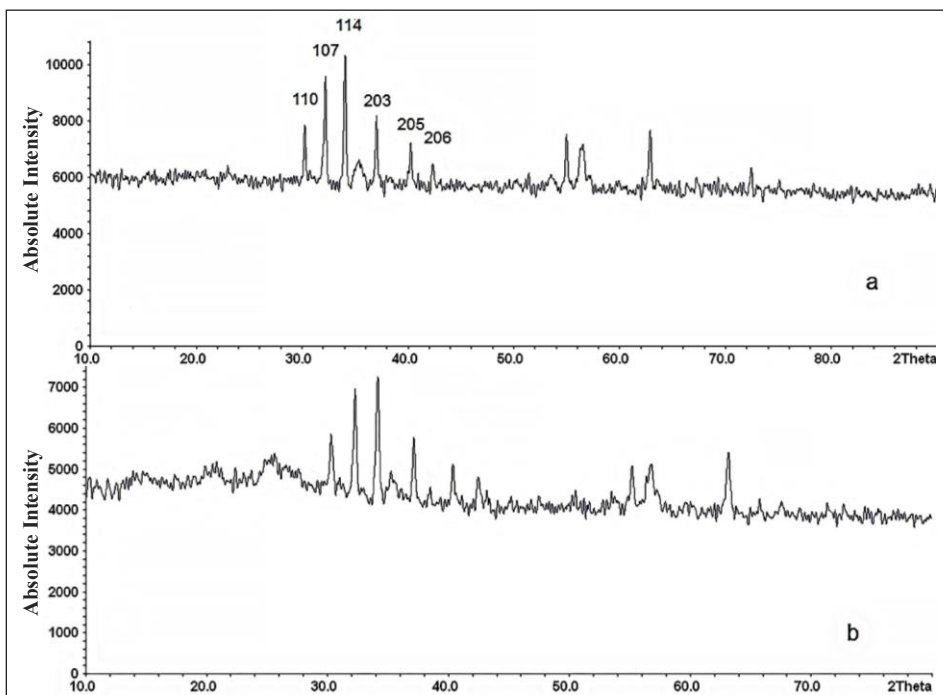
شکل ۱ الگوی XRD نمونه‌های \text{SrFe}_{11.1}(\text{Zn}_{0.5}\text{Co}_{0.5}\text{Zr})_{0.45}\text{O}_{19} (a) و نانوجندسازه پلی‌آنیلین/ \text{SrFe}_{11.1}(\text{Zn}_{0.5}\text{Co}_{0.5}\text{Zr})_{0.45}\text{O}_{19} (b)
