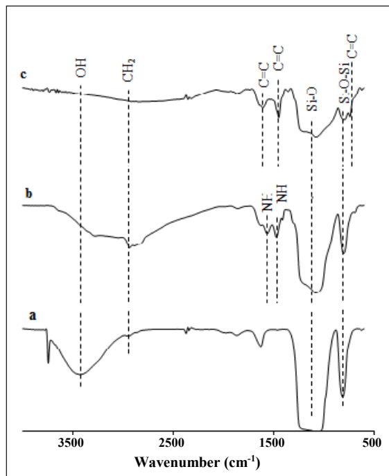
شکل ۳ طیف های فرورسوخ (a) T-SBA-15 و (b) SBA-15 و (c) FT-SBA-15
