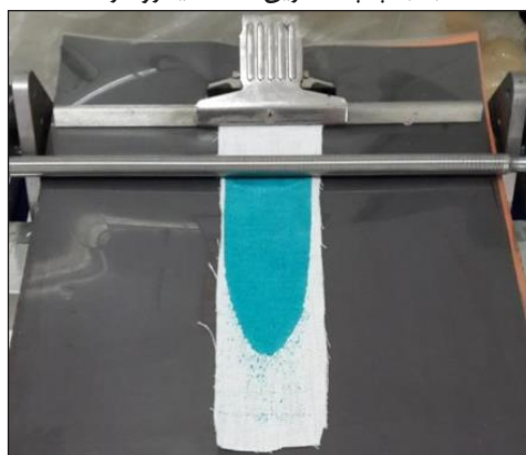
شکل ۲ چاپ خمیر میکروکپسول HD@MF بر پارچه
