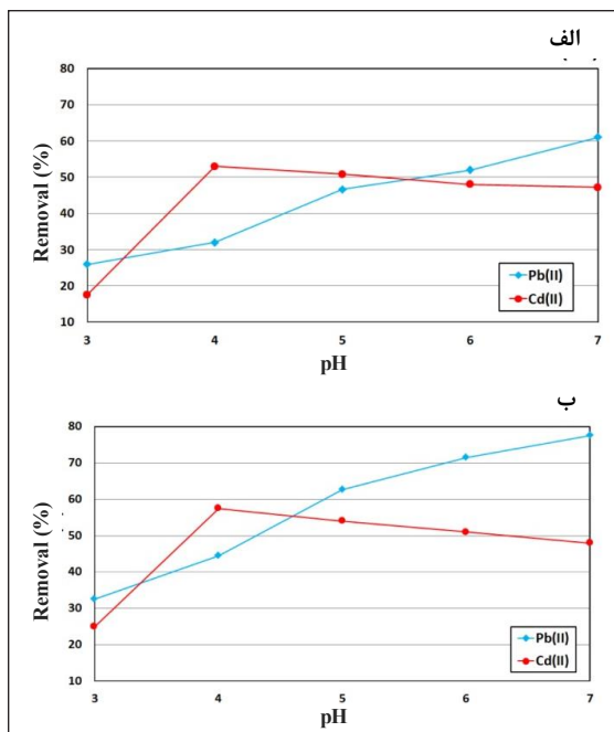
شکل ۵ اثر pH بر مقدار حذف سرب (II) و کادمیم با چندسازه‌های Zeolite N.P./HPC/GO (الف) و Zeolite N.P./GO (ب)
