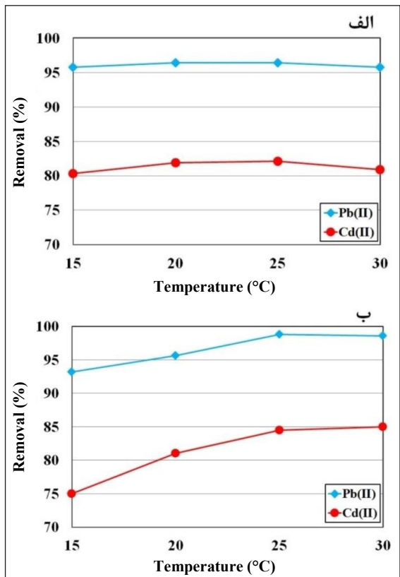
شکل ۸ اثر دما بر مقدار حذف یون‌های سرب (II) و کادمیم با چندسازه‌های Zeolite N.P./HPC/GO (الف) و Zeolite N.P./GO (ب)
