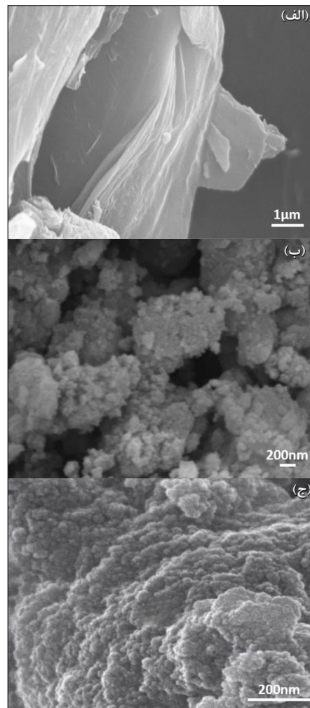
شکل ۱ تصاویر SEM گرافن اکسید (الف)، چندسازه (ب) Zeolite N.P./GO و چندسازه (ج) Zeolite N.P./HPC/GO
