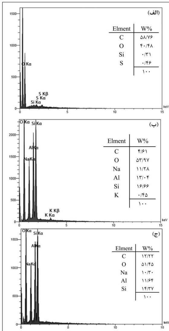
شکل ۲ طیف‌های EDS گرافن اکسید (الف)، چندسازه (ب) Zeolite N.P./GO و چندسازه (ج) Zeolite N.P./HPC/GO
