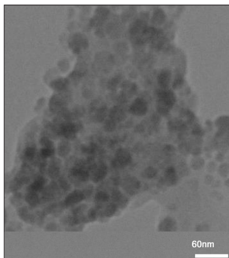
شکل ۴ تصویر TEM نانو کاتالیست Fe_3O_4 @CS-CS_{OX}@Pd
