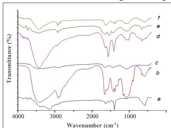
شکل ۵ طیف‌های FTIR کاتالیست Fe_3O_4 @CS-CS_{OX}@Pd آهن اکسید (a)، کیتوسان (b)، کیتوسان اکسید (c)، کیتوسان / کیتوسان اکسید (d)، کیتوسان / کیتوسان اکسید کاهش یافته (e) و Fe_3O_4 @CS-CS_{OX}@Pd (f)
