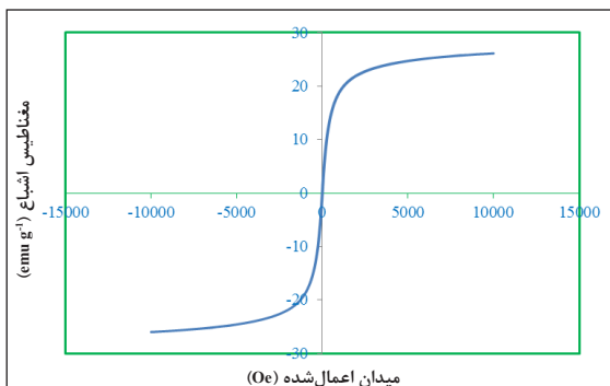
شکل ۸ تصویر VSM نانوکاتالیست Fe_3O_4 @CS-CS_{ox}@Pd
