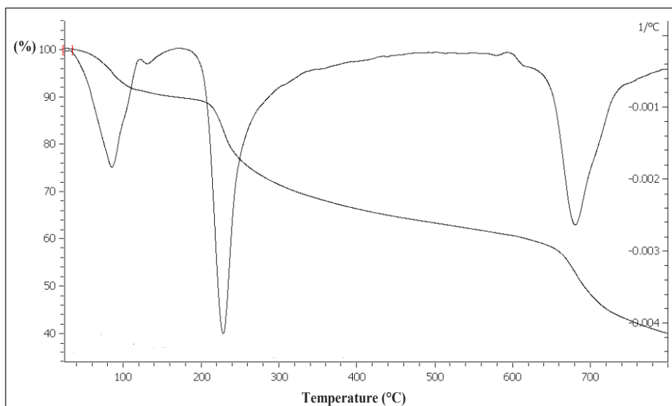
شکل ۹ TG-DTG نانوکاتالیست Fe_3O_4@CS-CS_{OX}@Pd
