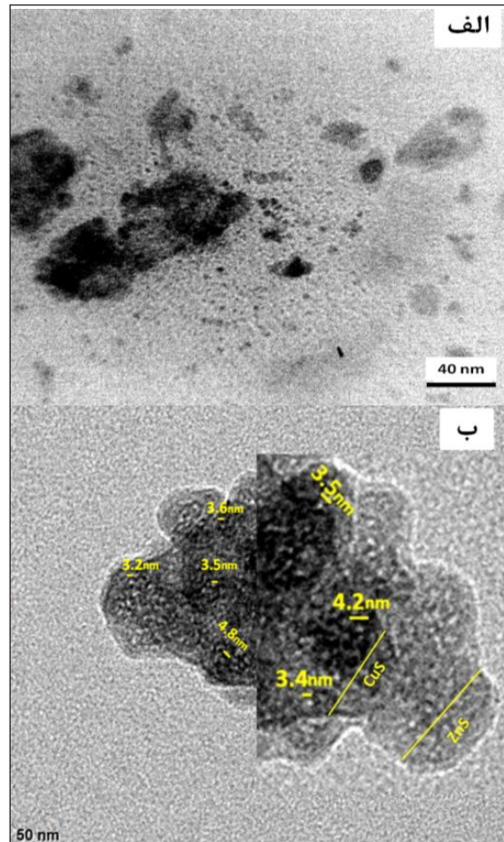
شکل ۳ تصویر TEM لایه نازک ZnS (الف) لایه نازک ZnS:CuS (ب) به‌دست آمده از غوطه‌ورسازی لایه نازک ZnS در محلول مس (II) کلرید با مدت‌های غوطه‌ورسازی ۱ دقیقه (بخش سمت راست شکل (ب) برای دید بهتر، بزرگ‌تر شده است).
