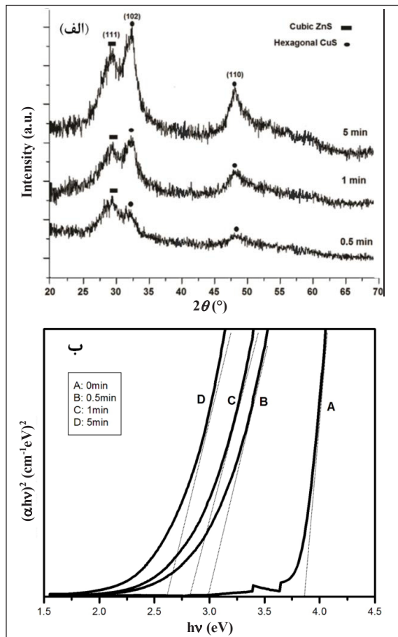
شکل ۱ الگوهای پراش پرتو ایکس لایه‌های نازک ZnS:CuS با زمان‌های غوطه‌ورسازی ۰٫۵، ۱ و ۵ دقیقه (الف) و نمودار (\alpha hv)^2 بر حسب hv (ب) مربوط به لایه‌های نازک ZnS:CuS متناظر با زمان‌های غوطه‌ورسازی (ZnS)، ۰٫۵، ۱ و ۵ دقیقه
