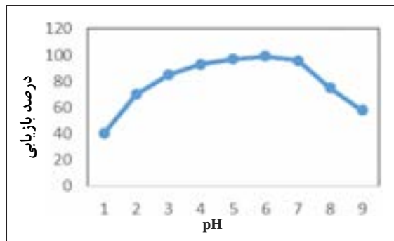
شکل ۱ اثر pH بر مقدار جذب نقره ( [Ag^+] = 6.66 \text{ mg l}^{-1} ، مقدار جاذب = ۰٫۰۵ g، pH=۶، حجم نمونه = ۳۰ ml)
