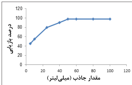
شکل ۱۲ بررسی مقدار فاز جامد بر استخراج یون نقره در روش ستون ( [Ag^+] = 1 \text{ mg l}^{-1} ، مقدار جاذب = 0.05 g، pH=6، حجم نمونه = 10 ml، حجم شوینده = 2 ml)
