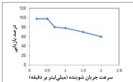
شکل ۱۰ تغییرات سرعت جریان نمونه بر جذب یون نقره (حجم نمونه = 10 ml، حجم شوینده = 2 ml، [Ag^+] = 0.5 \text{ mg l}^{-1} ، مقدار جاذب = 0.05 g، pH=6، حجم نمونه = 10 ml)
