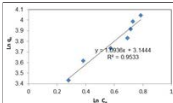
شکل ۸ بررسی جذب نقره با معادله فرندلیچ (مقدار لیگاند \Delta_3 = 10 \text{ mg l}^{-1} ، \text{pH} = 6 ) (مقدار جاذب g = 0.05 ، \text{pH} = 6 ، حجم نمونه = ۳۰ ml)
