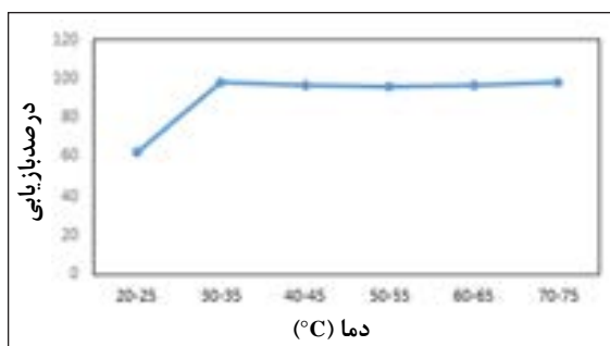
شکل ۴ بررسی اثر دما بر تهیه جاذب برای استخراج نقره (مقدار لیگاند = ۳ mg، [Ag^+] = 10 \text{ mg l}^{-1} ، مقدار جاذب = ۰٫۰۵ g، pH=۶، حجم نمونه = ۳۰ ml)
