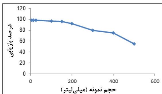
شکل ۱۱ تغییرات حجم نمونه بر درصد جذب یون نقره ( [Ag^+] = 1 \text{ mg l}^{-1} ، مقدار جاذب = 0.05 g، pH=6، حجم نمونه = 10 ml، حجم شوینده = 2 ml)
