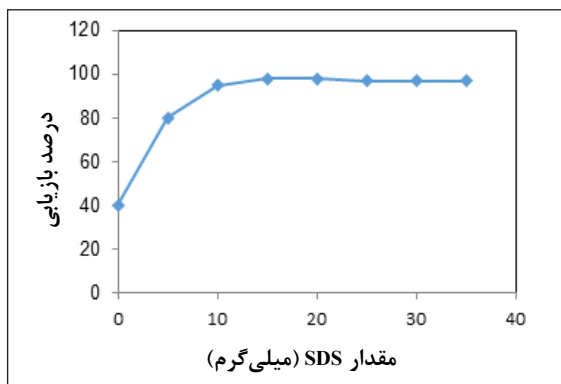
شکل ۳ بررسی اثر مقدار SDS بر مقدار جذب نقره (مقدار لیگاند = ۳ mg، [Ag^+] = 10 \text{ mg l}^{-1} ، مقدار جاذب = ۰٫۰۵ g، pH=۶، حجم نمونه = ۳۰ ml)
