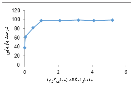
شکل ۲ اثر مقدار لیگاند بر مقدار جذب نقره (مقدار جاذب = ۰٫۰۵ g، pH=۶، [Ag^+] = 6.66 \text{ mg l}^{-1} ، حجم نمونه = ۳۰ ml)
