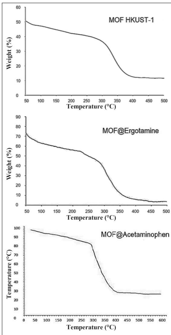
شکل ۵ نمودار آزمون وزنی گرمایی چارچوب آلی-فلزی HKUST-1 پیش و پس از بارگذاری داروها
