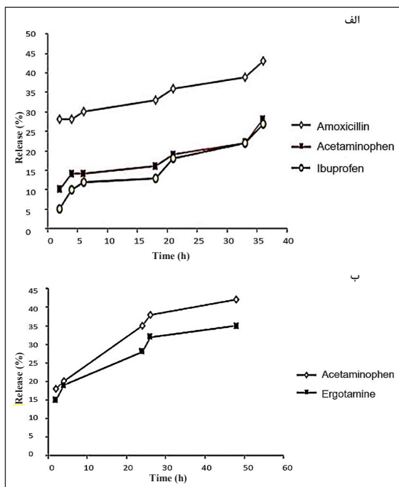
شکل ۶ رها سازی داروها از چارچوب آلی-فلزی UiO-66-NH 2 (الف) و HKUST-1 (ب)
