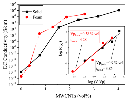
شکل ۶ رسانش الکتریکی DC و مدل توانی (پیوست تصویر) مربوط به نانوپندسازه‌های غیرمتخلخل و اسفنجی EPDM/MWCNT بر حسب درصد حجمی پرکننده MWCNT
